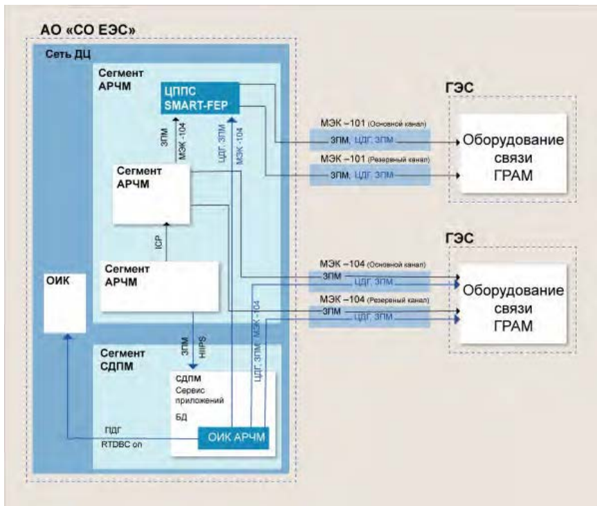
Структура СДПМ
