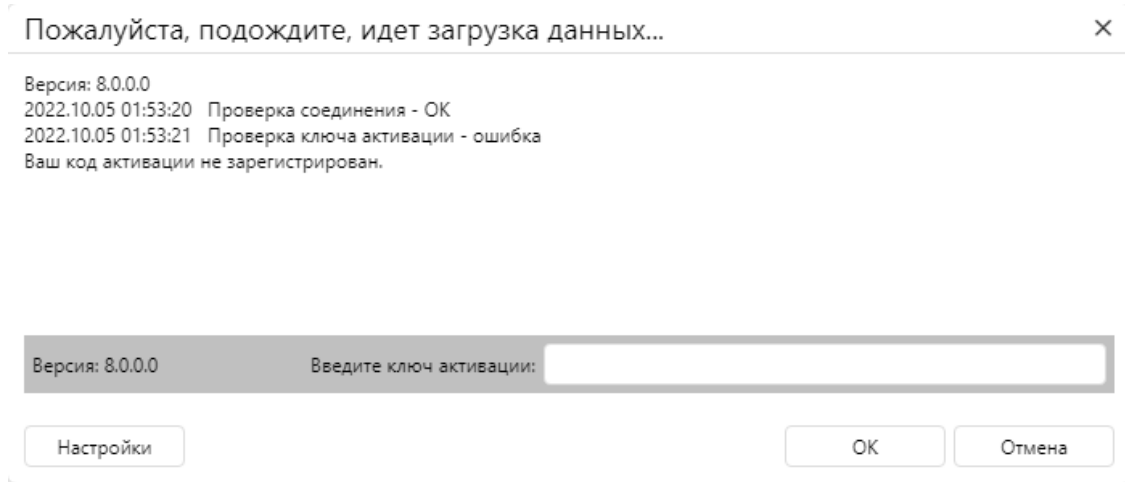
Рисунок 7.11 Предупреждающее сообщение
