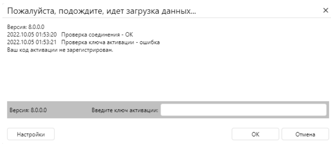
Рисунок 7.36 Предупреждающее сообщение
