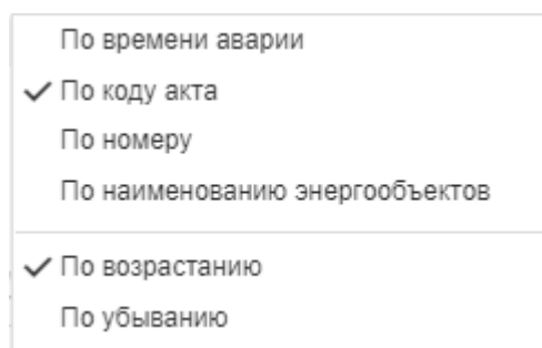
Рисунок 9.18 Функции сортировки
