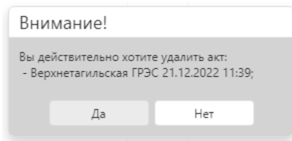
Рисунок 9.54 Предупреждающее сообщение
