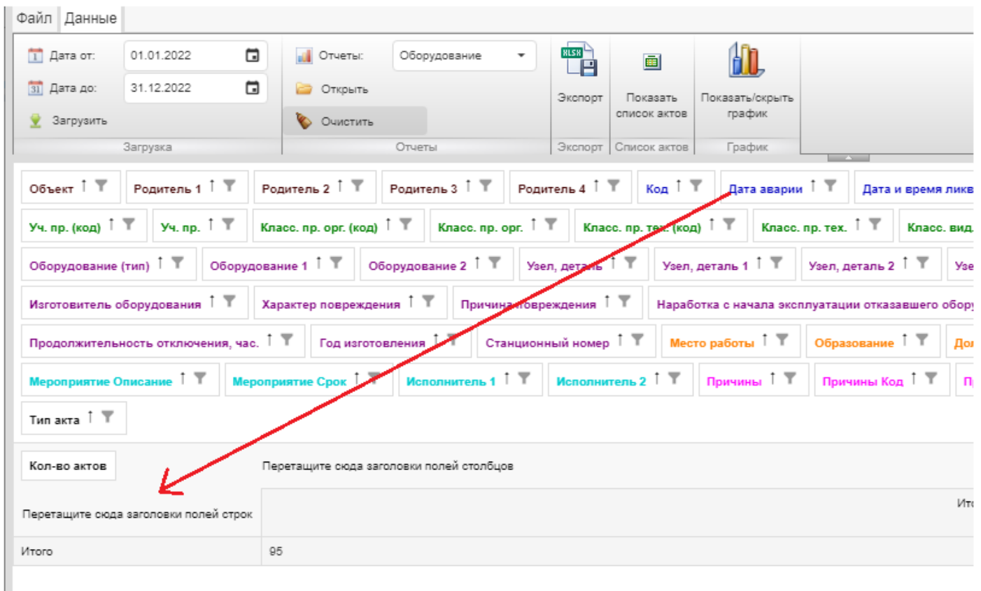
Рисунок 13.28 Перенос поля
