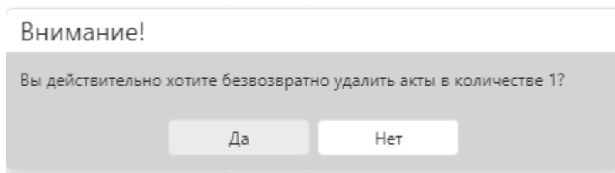
Рисунок 9.36 Предупредительное сообщение
