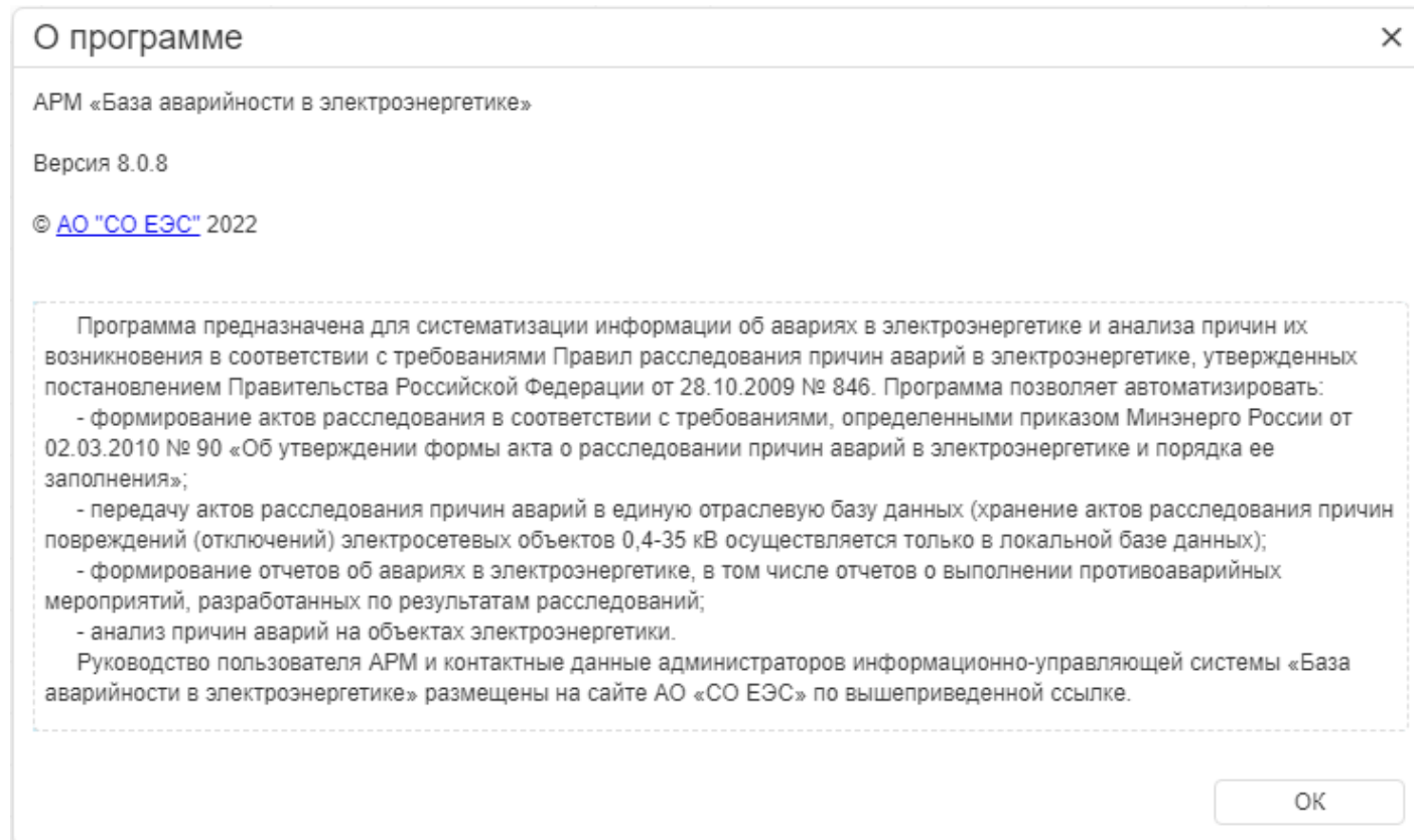
Рисунок 9.49 О программе
