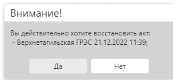
Рисунок 9.55 Предупреждающее сообщение
