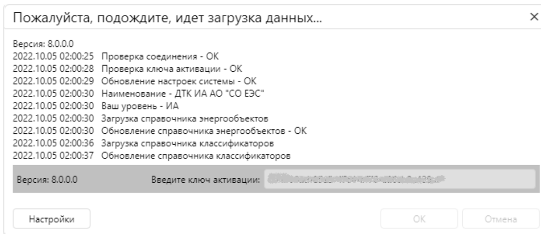
Рисунок 9.44 Окно инициализации
