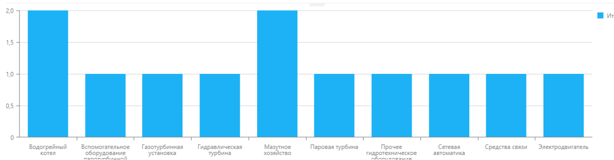
Рисунок 13.24 Гистограмма
