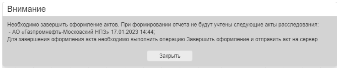
Рисунок 9.23 Предупреждающее сообщение
