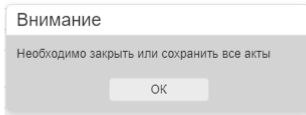
Рисунок 9.35 Предупредительное сообщение
