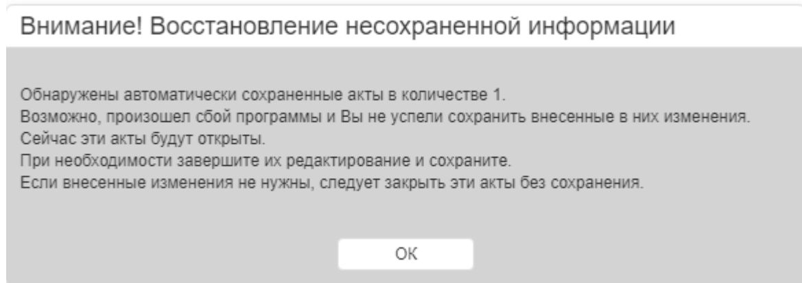
Рисунок 9.47 Предупреждающее сообщение
