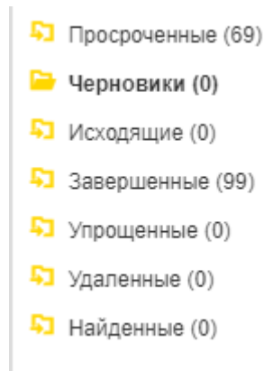
Рисунок 9.3 Зона папок
