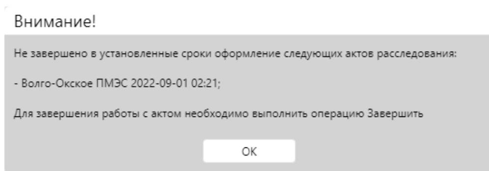
Рисунок 9.2 Информационное сообщение
