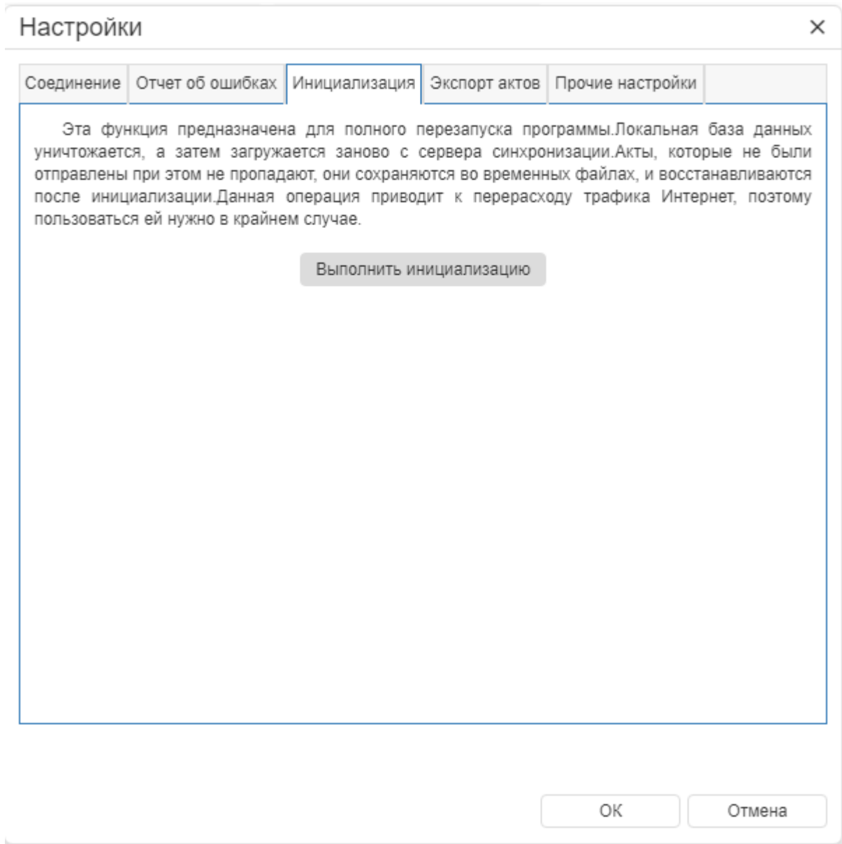
Рисунок 9.41 Вкладка инициализация
