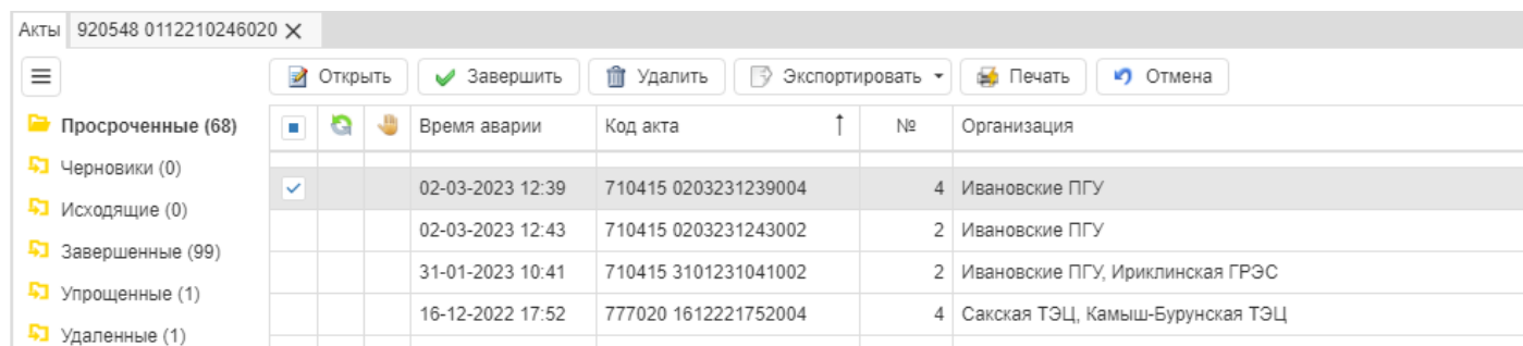
Рисунок 9.13 Выделенный акт
