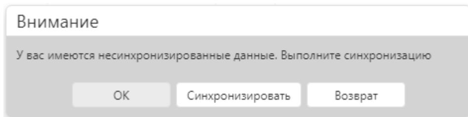
Рисунок 9.48 Предупреждающее сообщение
