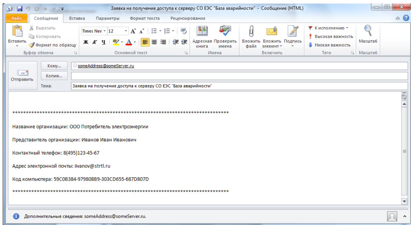
Рисунок 6.4 Отправка заявки
