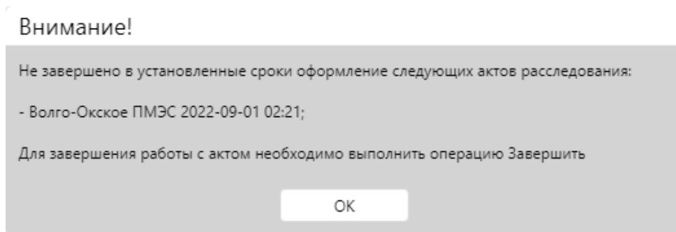
Рисунок 9.2 Информационное сообщение
