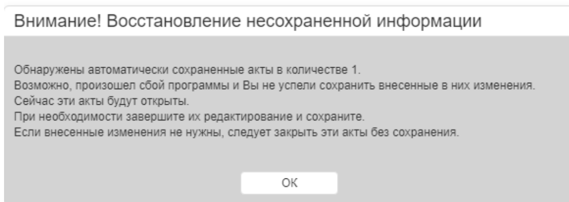
Рисунок 9.47 Предупреждающее сообщение
