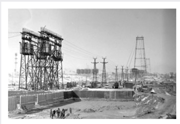
Строительство Сталинградской ГЭС. 1965 год
