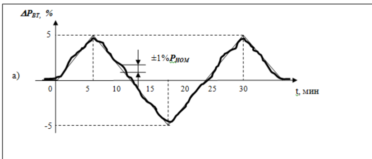
Рис.П.9. Имитация изменений задания и требуемые изменения вторичной мощности энергоблока при скорости задания изменения мощности 1\% P_{НОМ}/\text{мин}
