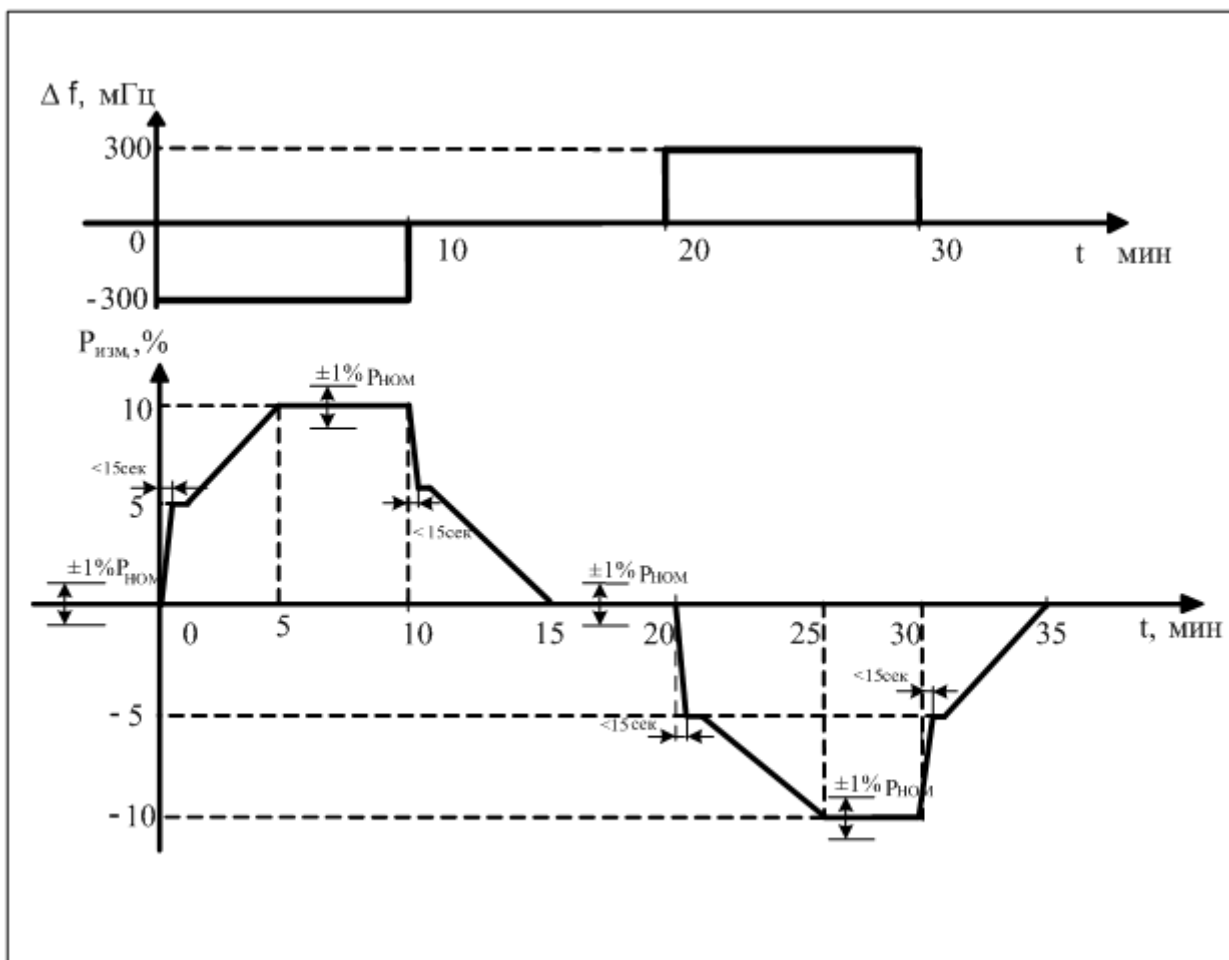
Рис.П.8 Имитация отклонений частоты и требуемые изменения первичной мощности энергоблока, работающего на газе при \Delta P_{П} = \pm 10\% P_{НОМ}
