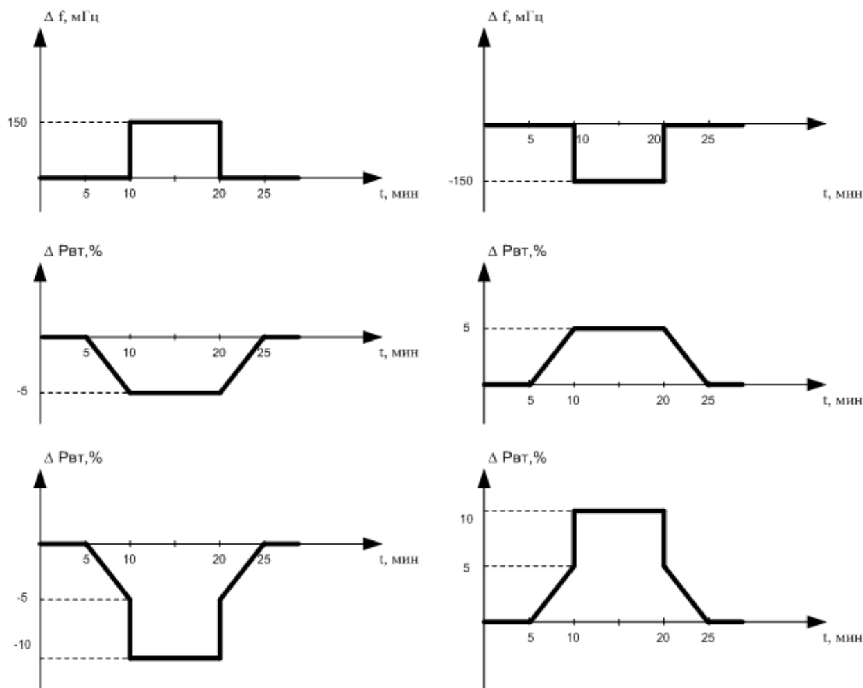
Рис.П.11. Имитация изменений задания вторичной мощности и отклонений частоты вниз (а) и вверх (б) регулировочного диапазона энергоблока
