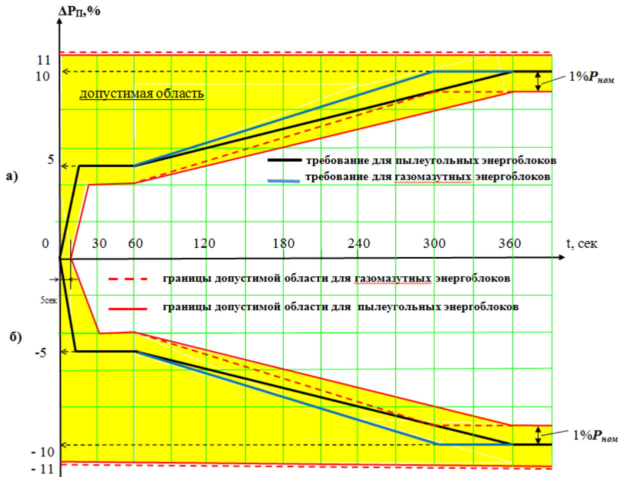
Рис.П.2. Допустимая область изменения первичной мощности энергоблока при \Delta P_{\text{п}} = \pm 10\% P_{\text{ном}} при снижении (а) и повышении (б) частоты
