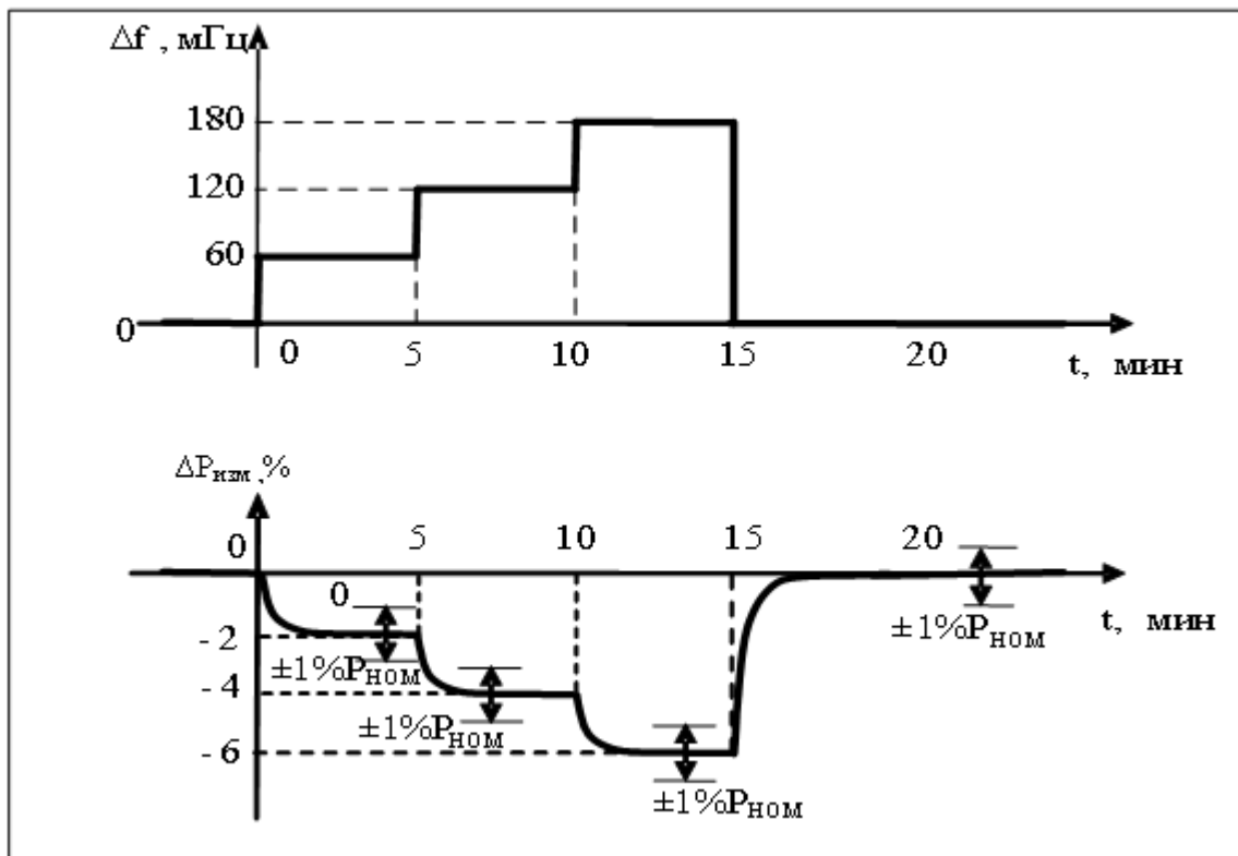
Рис.П.6. Имитация повышения частоты и требуемые изменения первичной мощности энергоблока в следящем режиме
