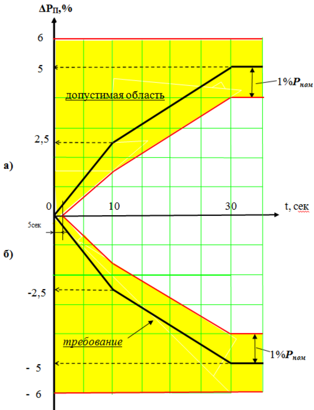
Рис.П.3. Допустимая область изменения первичной мощности энергоблока при \Delta P_{\text{П}} = \pm 5\%
