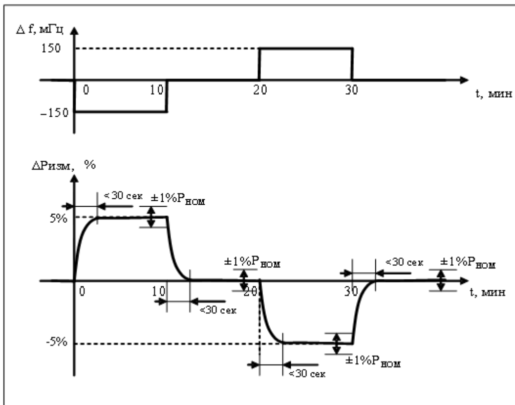
Рис.П.7. Имитация отклонений частоты и требуемые изменения первичной мощности энергоблока при \Delta P_{\Pi} = \pm 5\% P_{НОМ}
