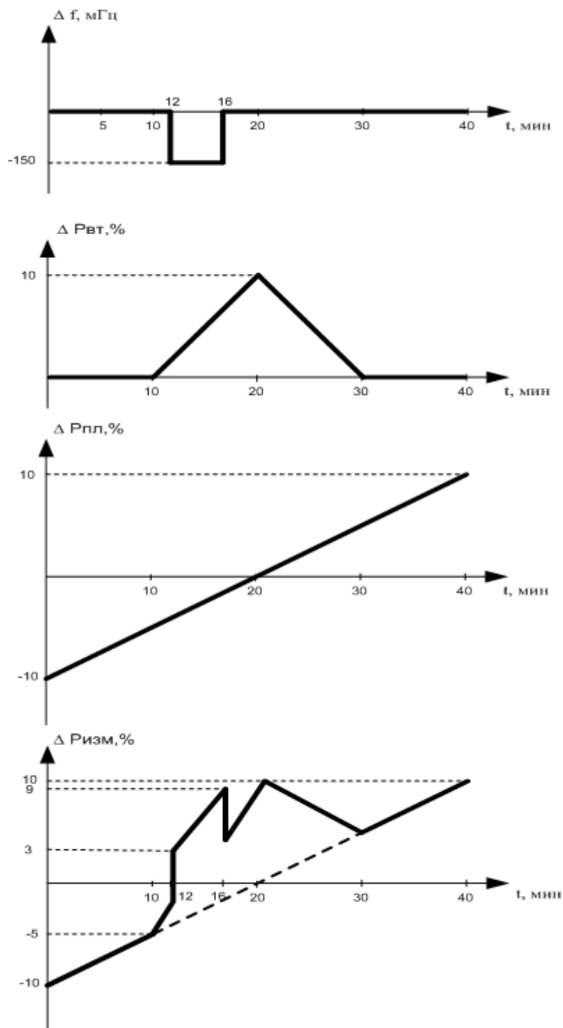
Рис.П.12. Имитация изменений заданий вторичной мощности и отклонений частоты при изменении планового задания энергоблока
