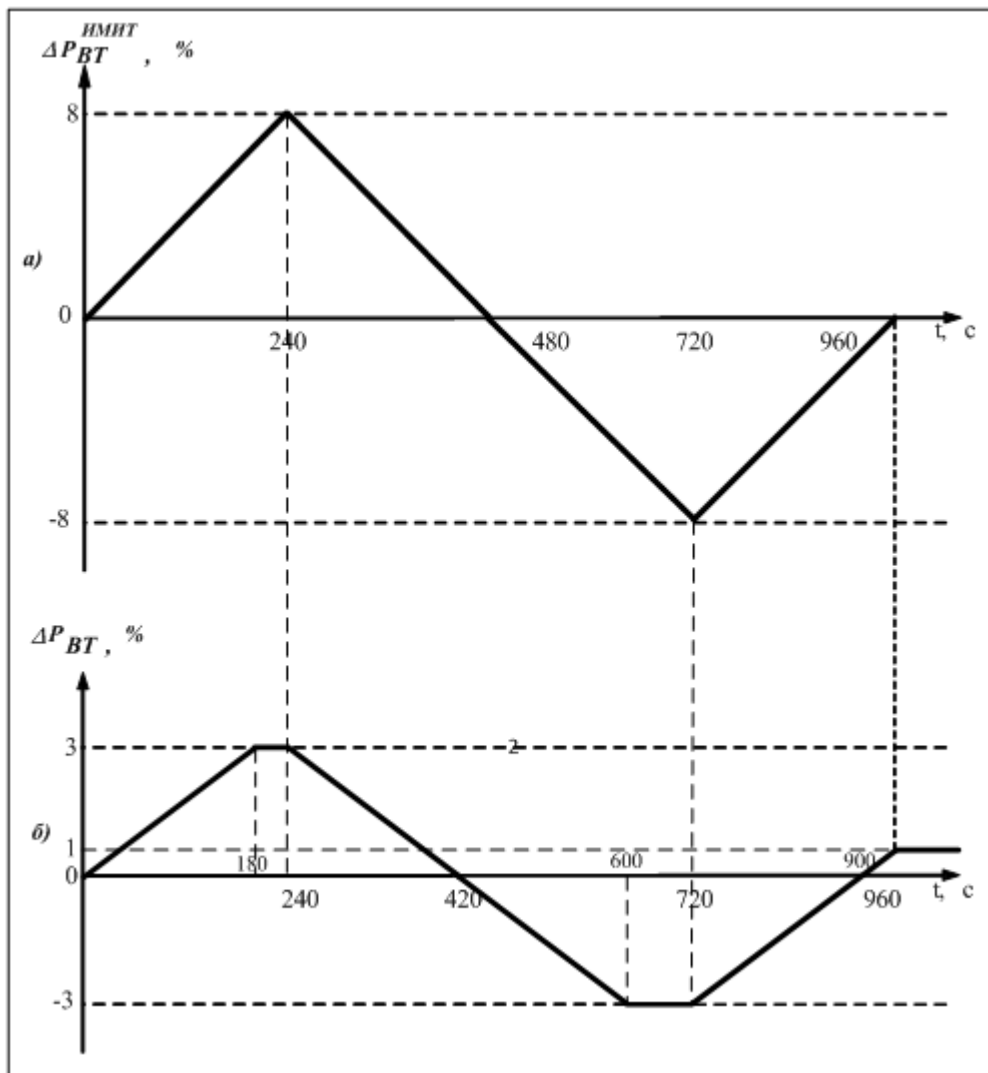
Рис.П.10. Имитация изменений задания \Delta P_{BT} = \pm 8\% P_{НОМ} со скоростью 2\% P_{НОМ}/\text{мин} (а) и требуемые изменения мощности энергоблока при установленных в САУМ ограничениях скорости и величин задания вторичной мощности соответственно 1\% P_{НОМ}/\text{мин} и \Delta P_{BT} = \pm 3\% P_{НОМ} (б)
