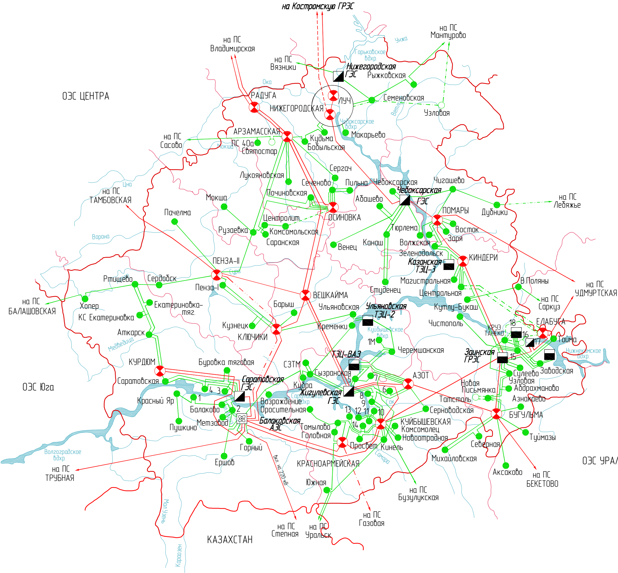
Карта-схема размещения линий электропередачи, подстанций напряжением 220 кВ и выше и электростанций ОЭС Средней Волги на 2014–2020 годы
