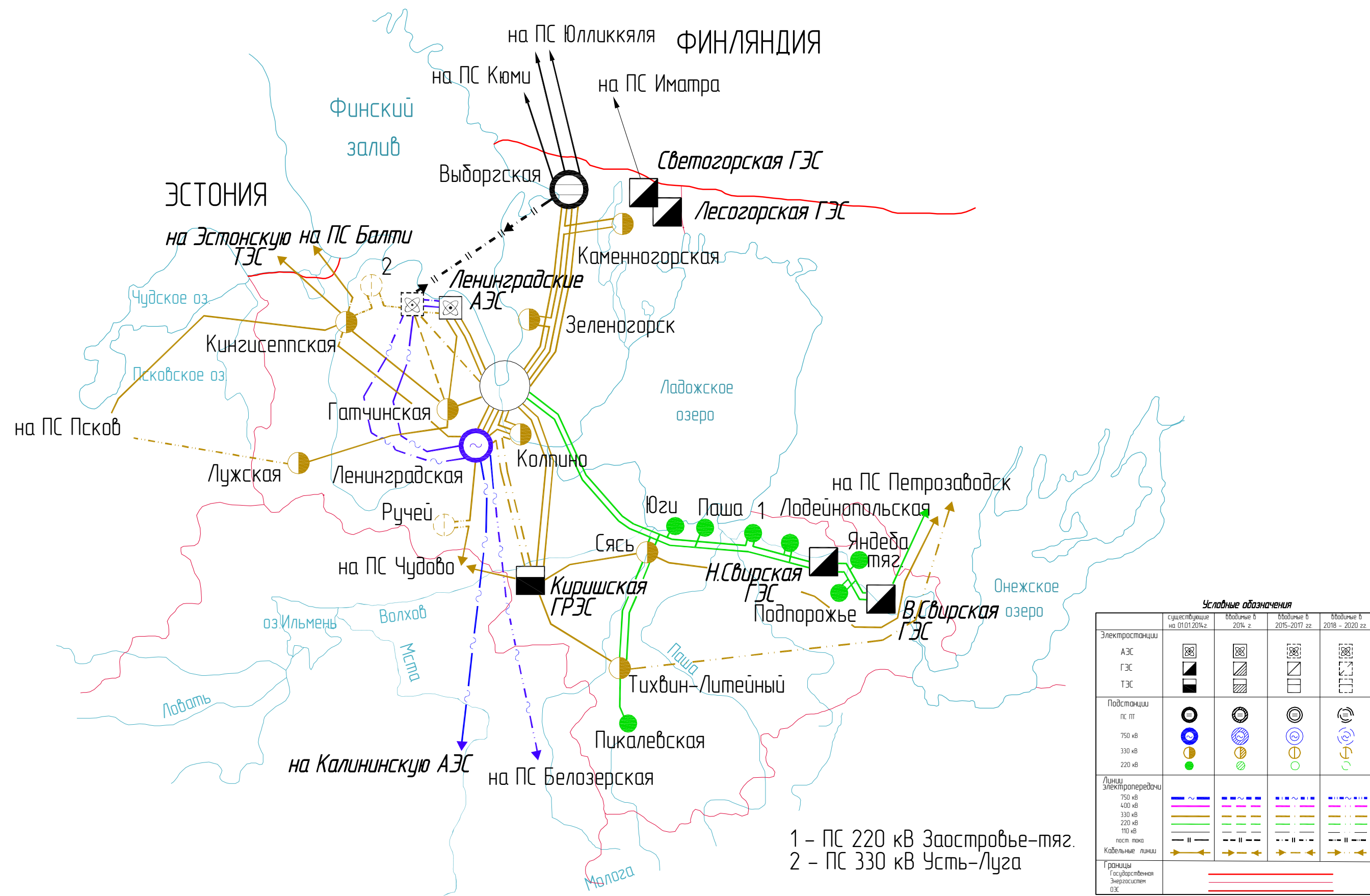
Карта-схема размещения линий электропередачи, подстанций напряжением 220 кВ и выше и электростанций Ленинградской энергосистемы на 2014–2020 годы
