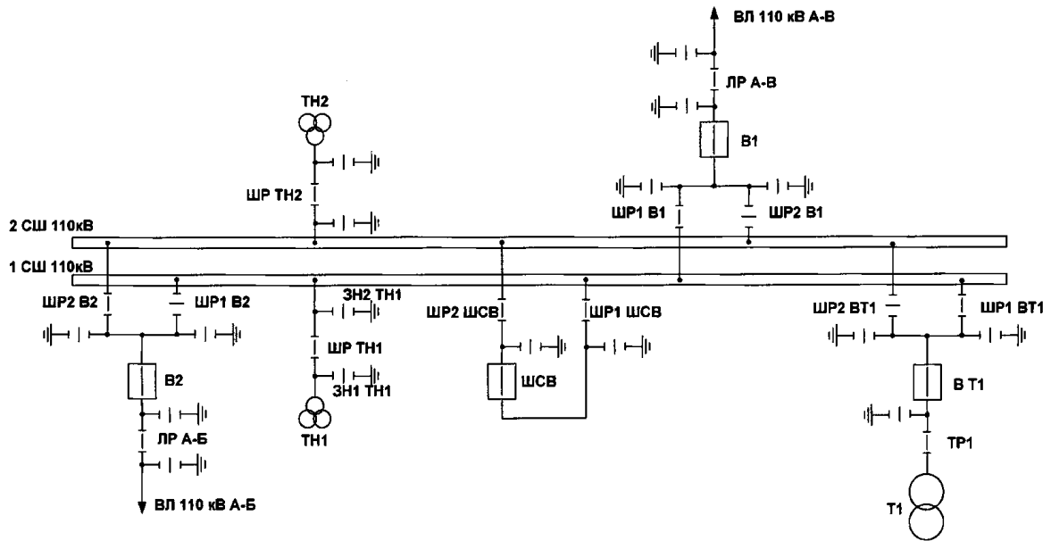
Рисунок 1. Схема РУ с двумя системами шин
