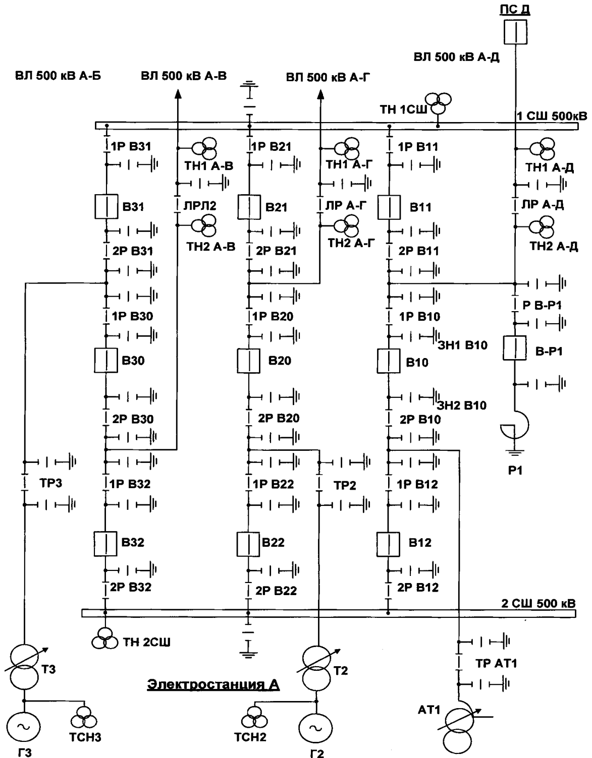
Рисунок 4. Полторная схема РУ
