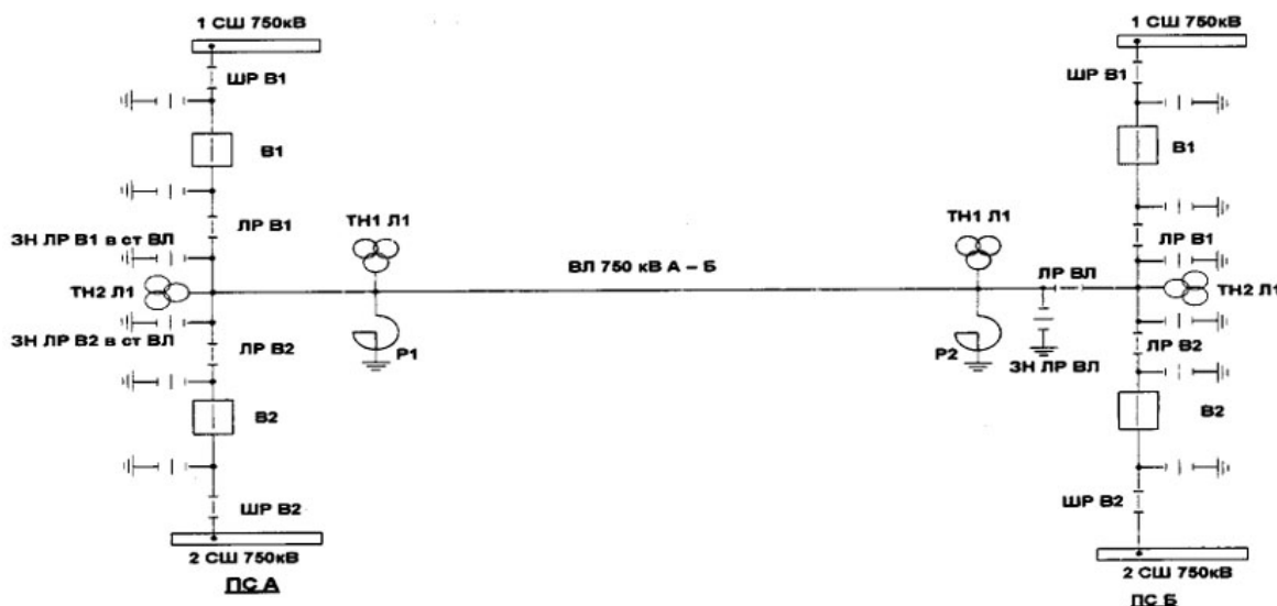
Рисунок 3-1. Схема подключения ВЛ 750 кВ А-Б
