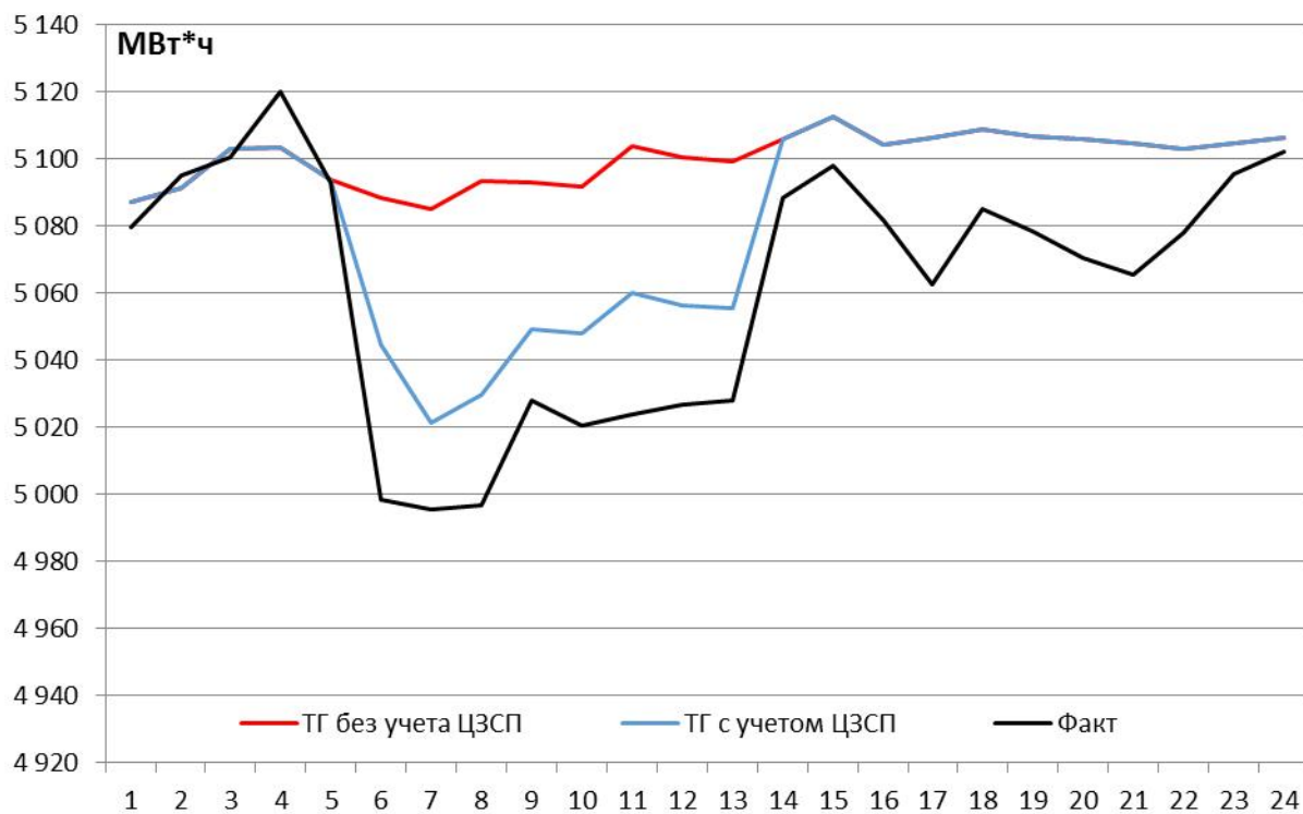
Рисунок 1 – Сводная информация по режиму работы потребителей с ЦЗСП
