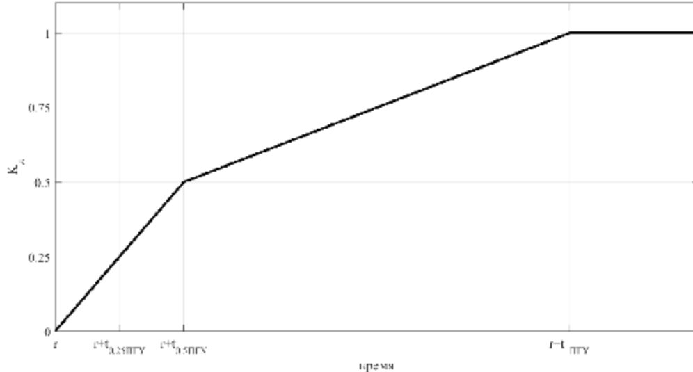
Рисунок 6. Коэффициент динамики для ПГУ
