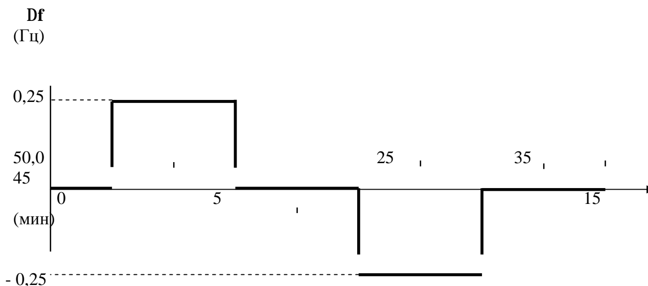
Рис.П.3.2.Порядок нанесения возмущений по частоте вращения в одной серии опытов при испытаниях (статизм 5 %)
