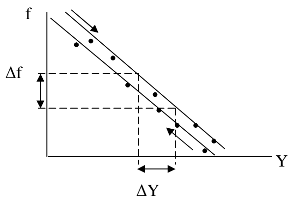
Статическая характеристика регулятора
