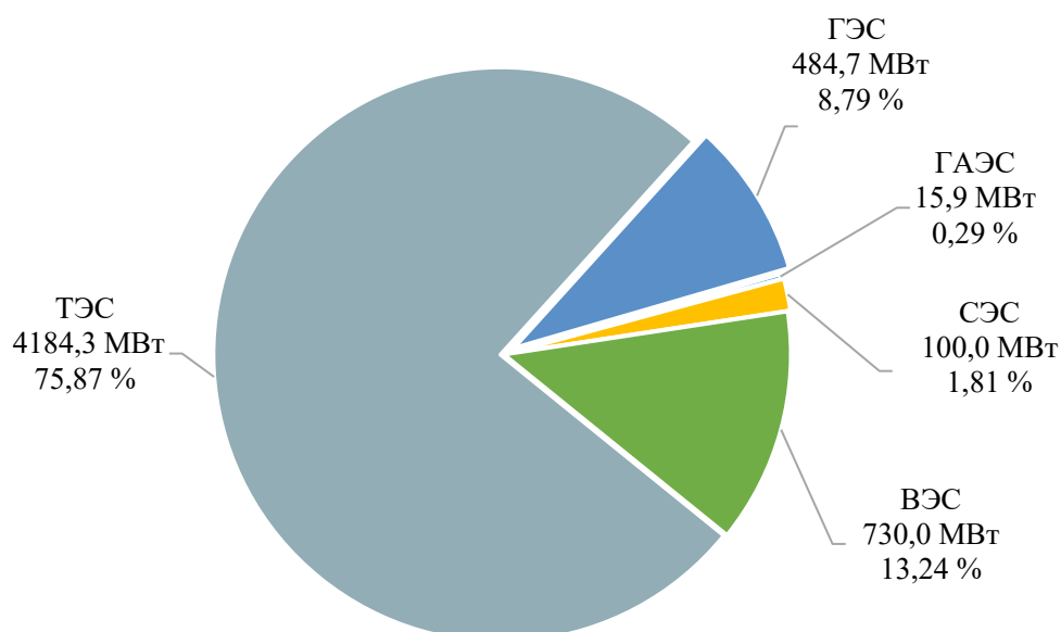
Рисунок 1 – Структура установленной мощности электростанций энергосистемы Ставропольского края по состоянию на 01.01.2024
