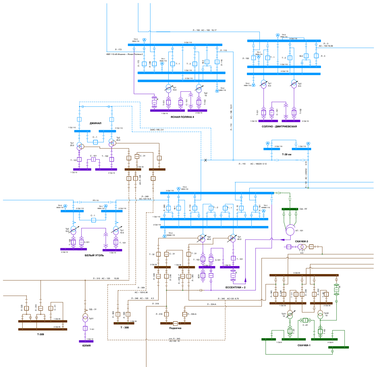
Рисунок 5 – Нормальная схема соединений электрической сети 35–110 кВ рассматриваемого района с реализованными мероприятиями варианта № 2
