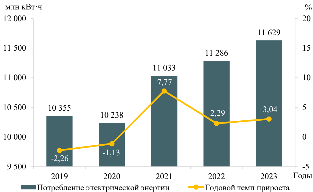
Рисунок 3 – Потребление электрической энергии энергосистемы Ставропольского края и годовые темпы прироста
