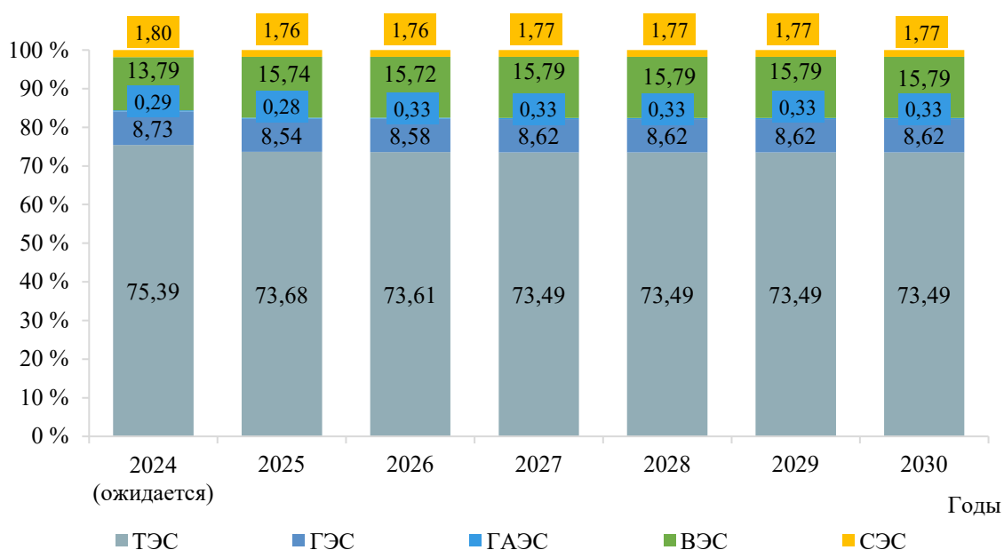
Рисунок 8 – Структура установленной мощности электростанций энергосистемы Ставропольского края
