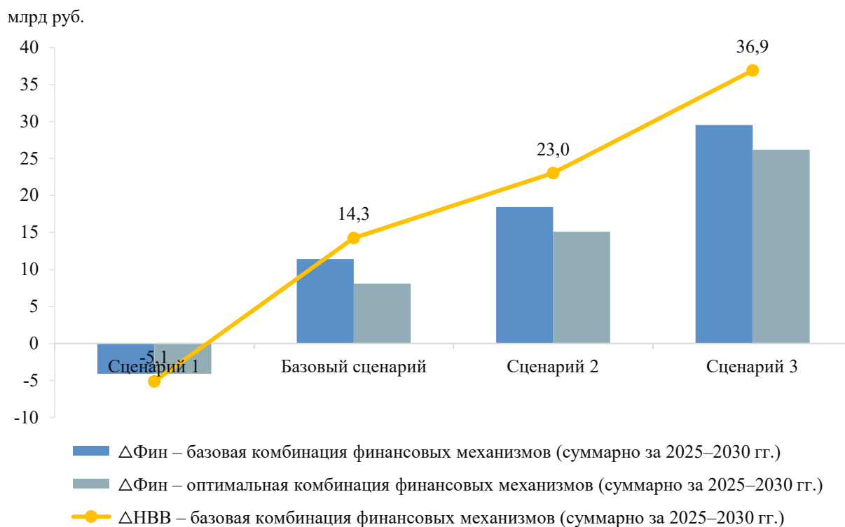
Рисунок 10 – Оценка чувствительности экономических условий реализации планируемого состава технических решений, предлагаемых к включению в схему и программу развития электроэнергетических систем России, от изменения темпов роста единого (котлового) тарифа на услуги по передаче электрической энергии на территории Ставропольского края
