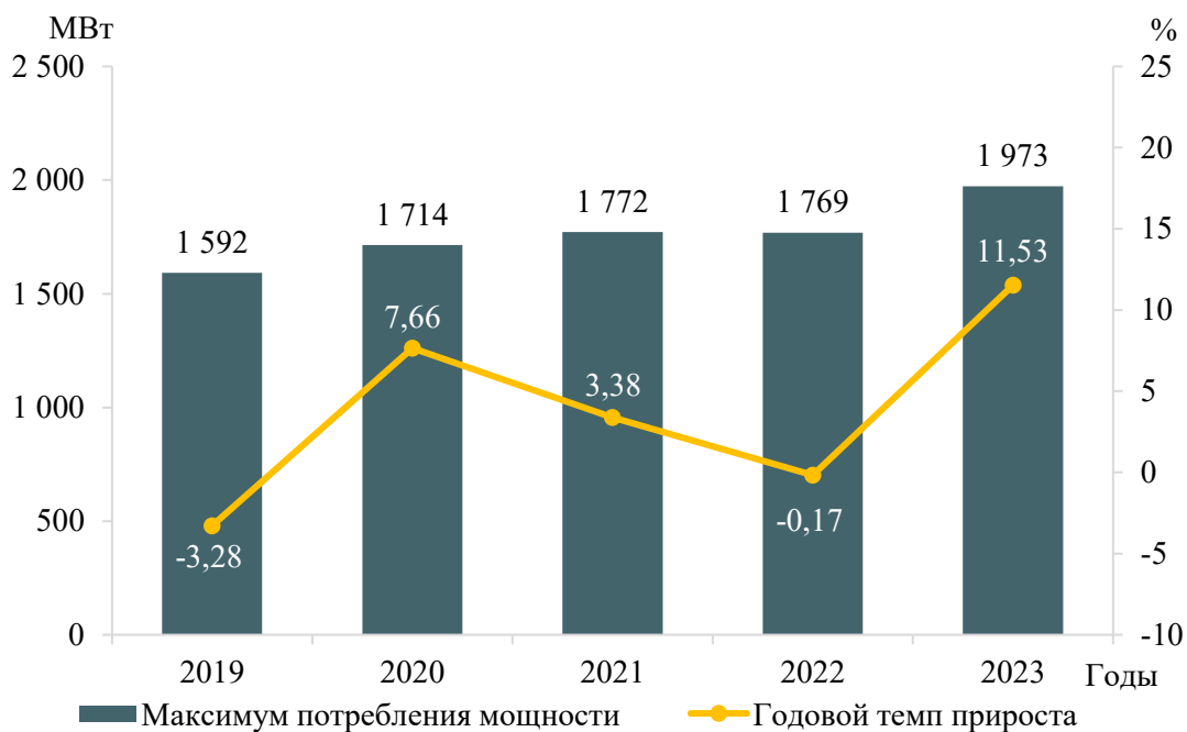
Рисунок 4 – Максимум потребления мощности энергосистемы Ставропольского края и годовые темпы прироста
