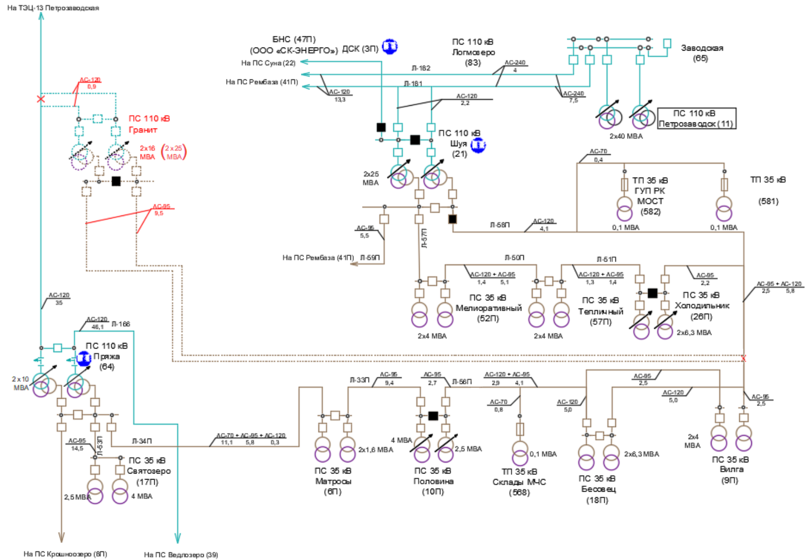
Рисунок 9 – Принципиальная схема района 35 кВ ПС 110 кВ Пряжа (ПС 64) – ПС 110 кВ Шuya (ПС 21) по варианту № 2
