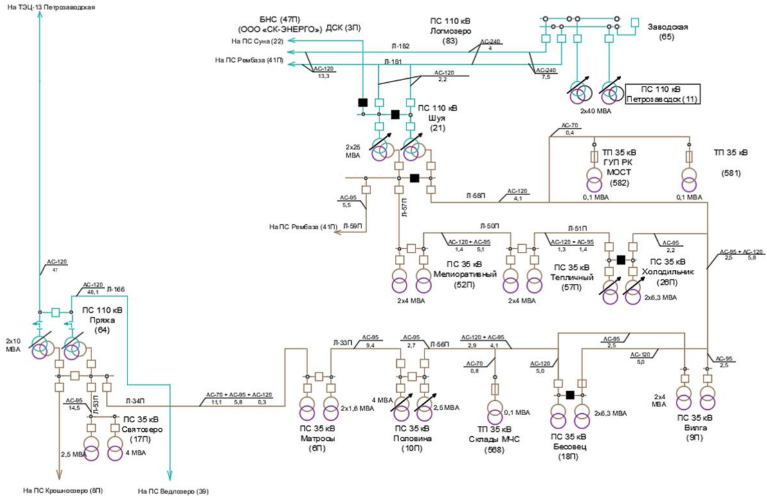
Рисунок 7 – Принципиальная схема района 35 кВ ПС 110 кВ Пряжа (ПС 64) – ПС 110 кВ Шуя (ПС 21)
