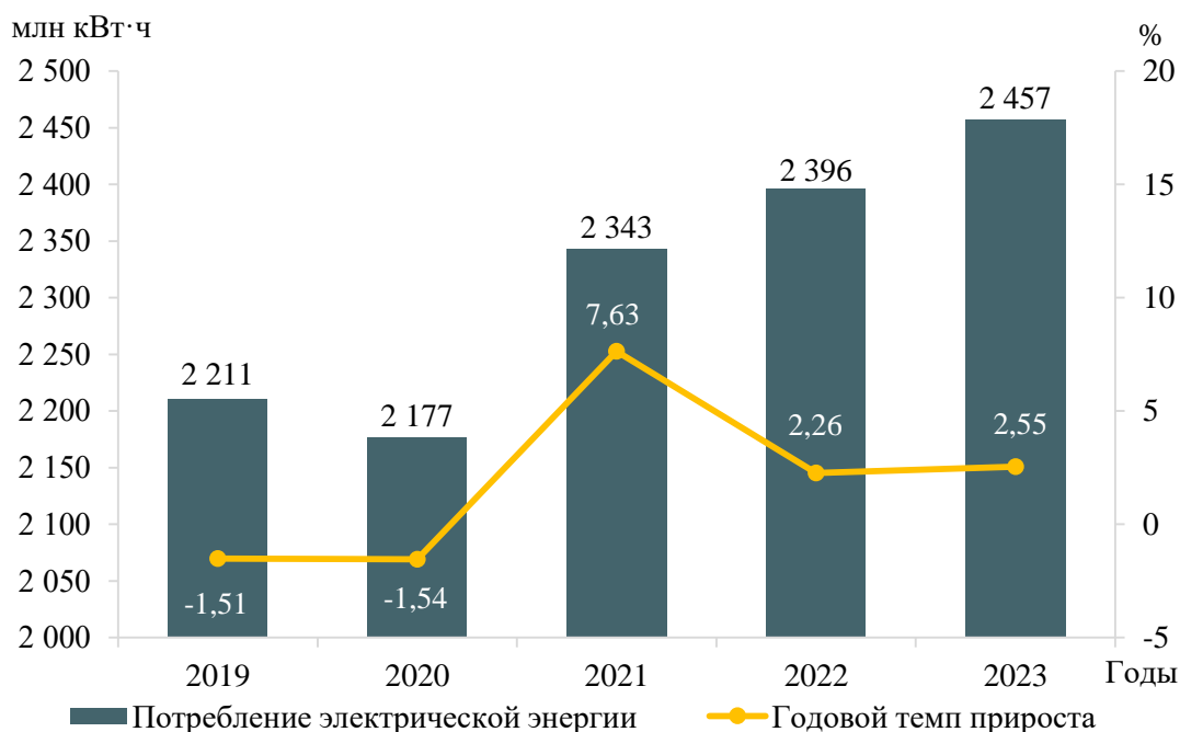
Рисунок 3 – Потребление электрической энергии энергосистемы Псковской области и годовые темпы прироста
