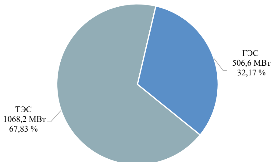
Рисунок 1 – Структура установленной мощности электростанций энергосистемы Ярославской области по состоянию на 01.01.2024
