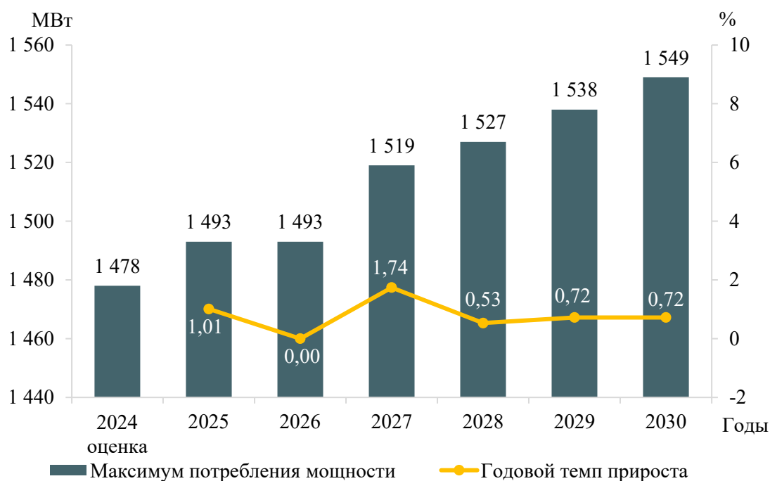
Рисунок 6 – Прогноз максимума потребления мощности энергосистемы Ярославской области и годовые темпы прироста
