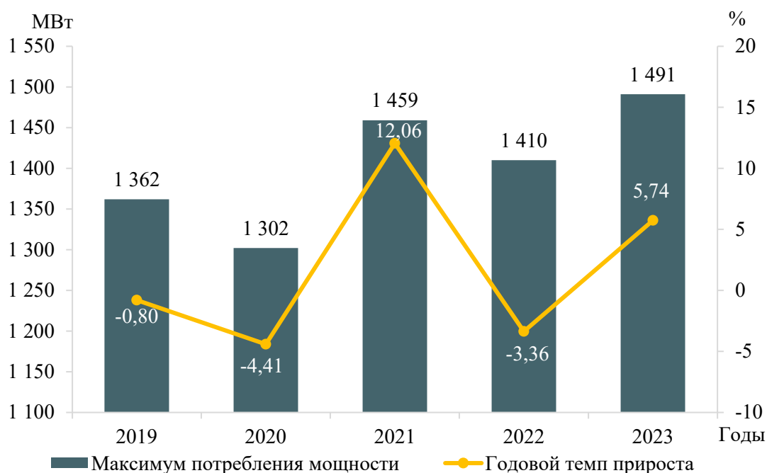
Рисунок 4 – Максимум потребления мощности энергосистемы по Ярославской области и годовые темпы прироста
