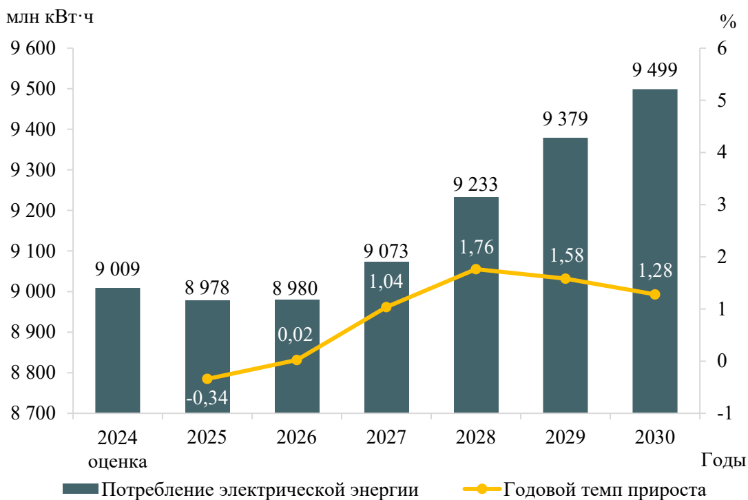
Рисунок 5 – Прогноз потребления электрической энергии энергосистемы Ярославской области и годовые темпы прироста
