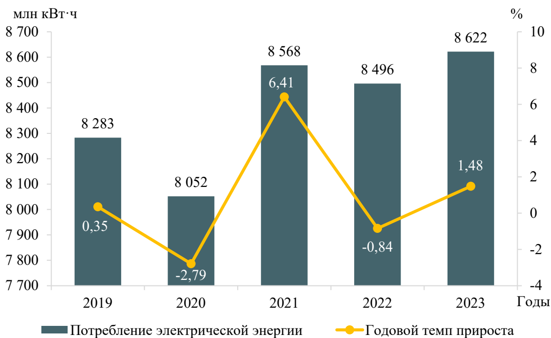
Рисунок 3 – Потребление электрической энергии энергосистемы Ярославской области и годовые темпы прироста
