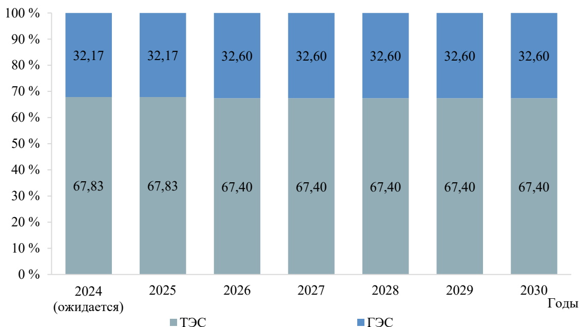
Рисунок 7 – Структура установленной мощности электростанций энергосистемы Ярославской области
