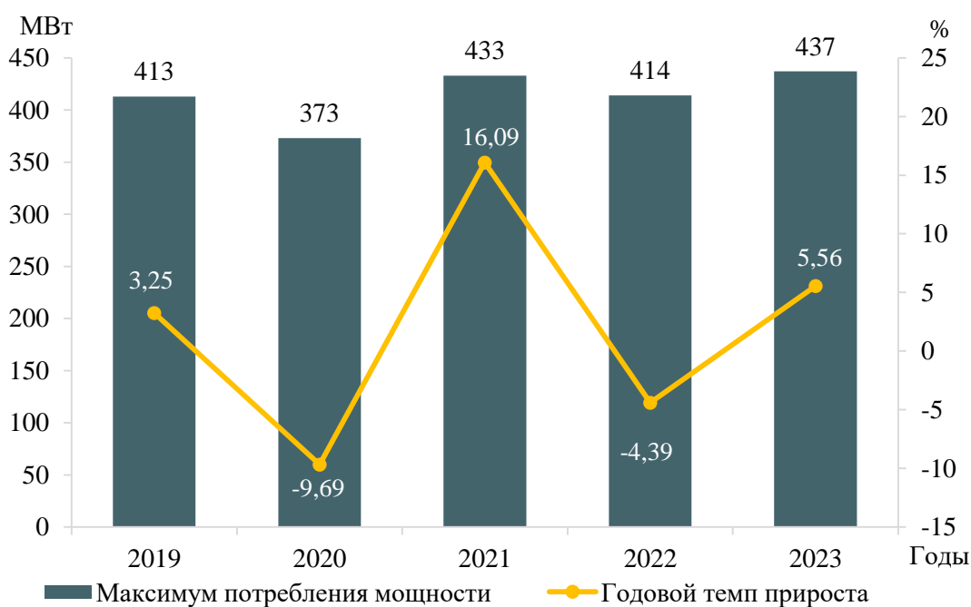
Рисунок 4 – Максимум потребления мощности энергосистемы Псковской области и годовые темпы прироста
