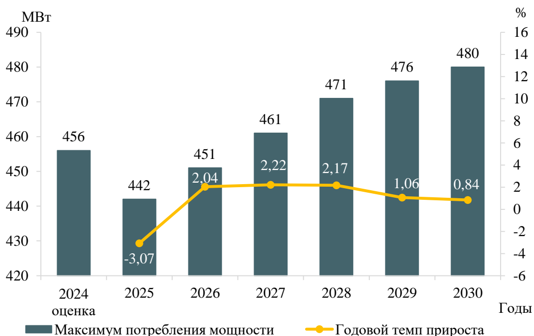
Рисунок 6 – Прогноз максимума потребления мощности и годовые темпы прироста энергосистемы Псковской области
