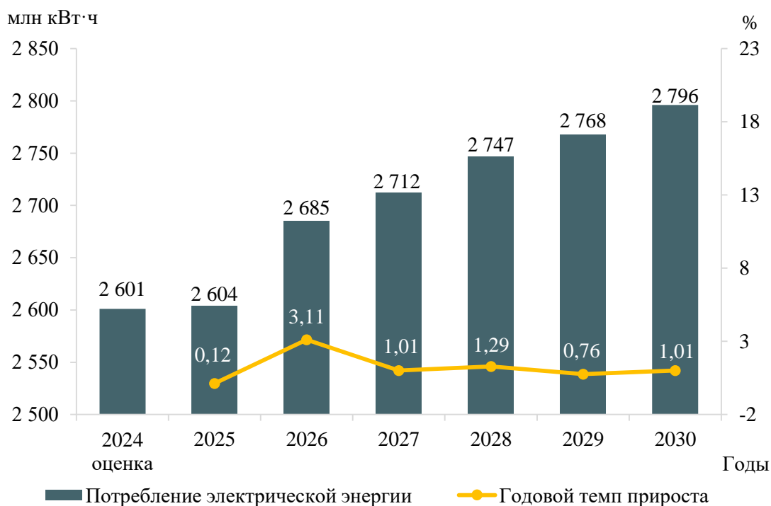
Рисунок 5 – Прогноз потребления электрической энергии энергосистемы Псковской области и годовые темпы прироста
