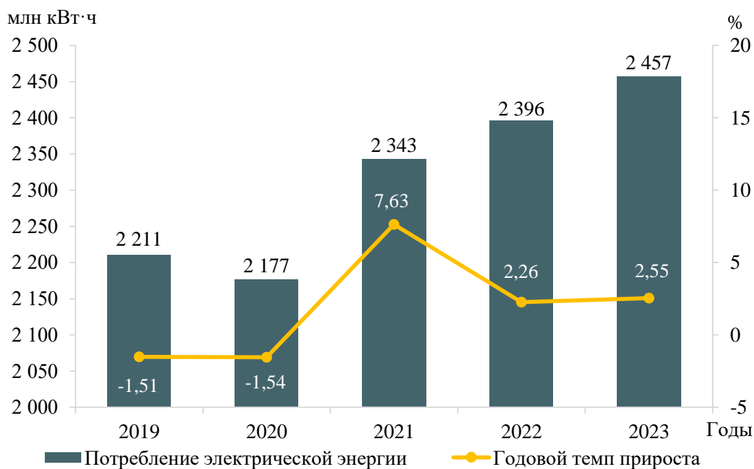
Рисунок 3 – Потребление электрической энергии энергосистемы Псковской области и годовые темпы прироста
