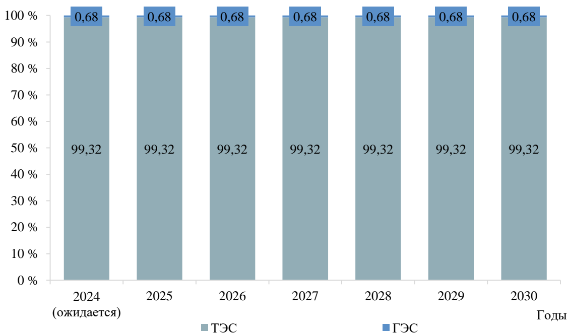
Рисунок 7 – Структура установленной мощности электростанций энергосистемы Псковской области
