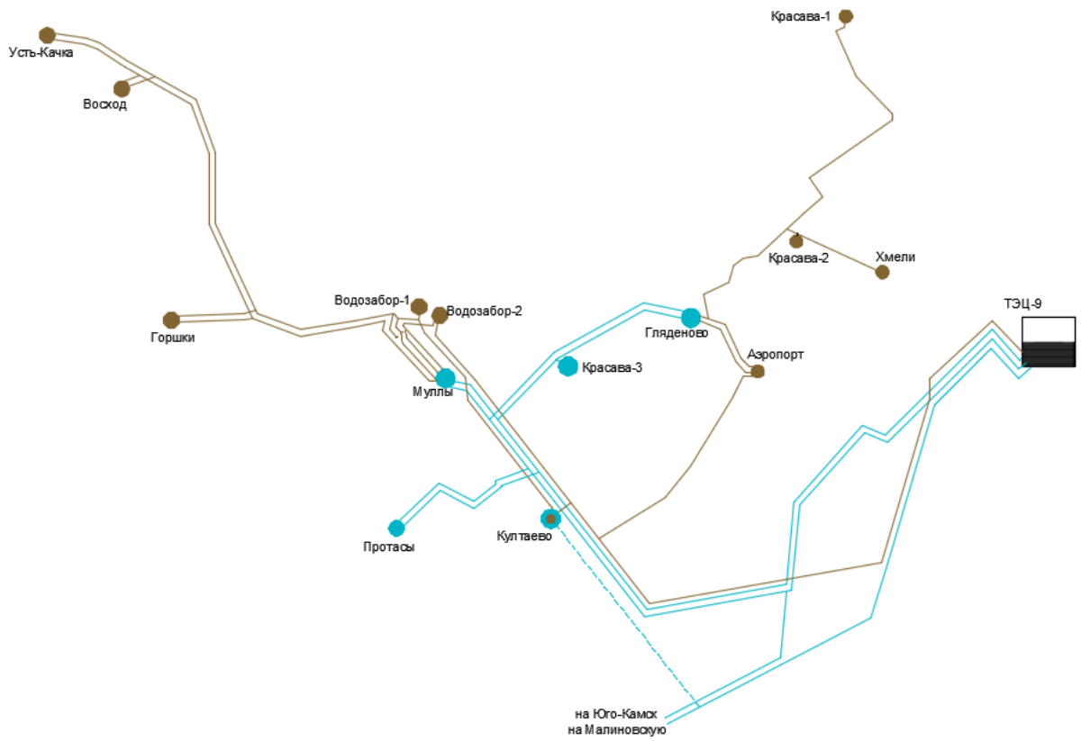
Рисунок 7 – Схема развития электрической сети 35–110 кВ рассматриваемого энергорайона по варианту № 1
