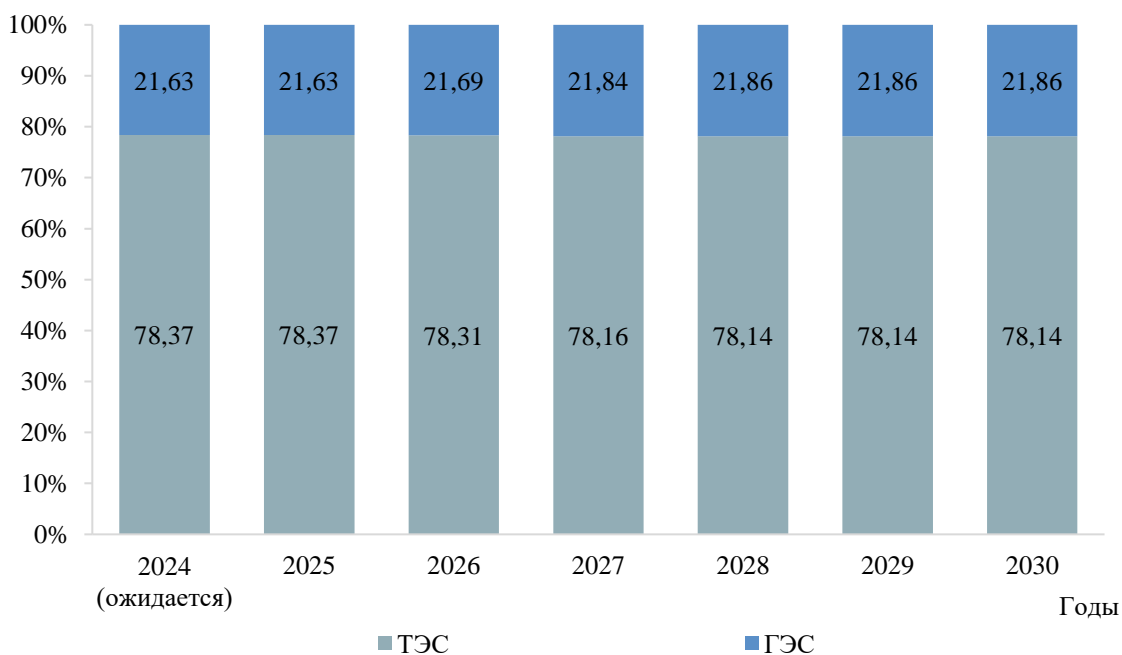
Рисунок 11 – Структура установленной мощности электростанций энергосистемы Пермского края
