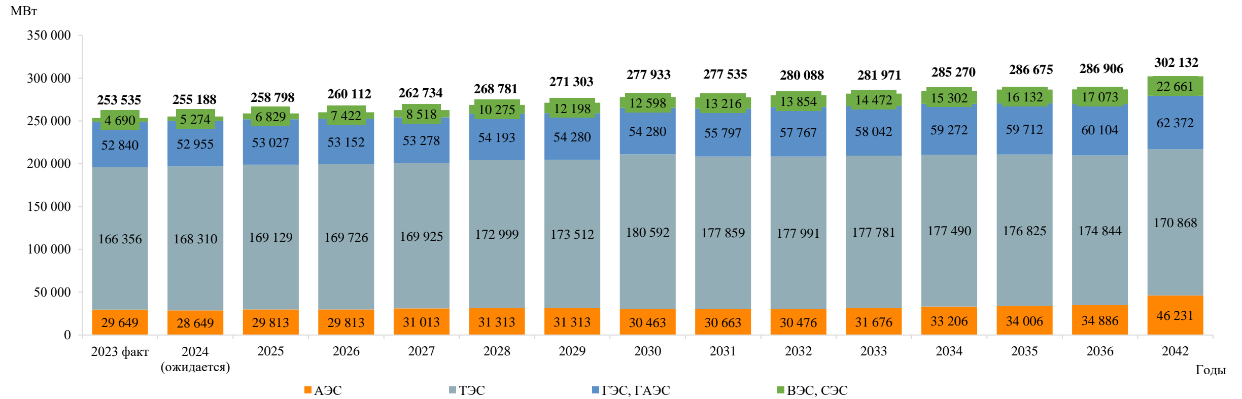
Рисунок 37 – Установленная мощность на электростанциях электроэнергетических систем России
