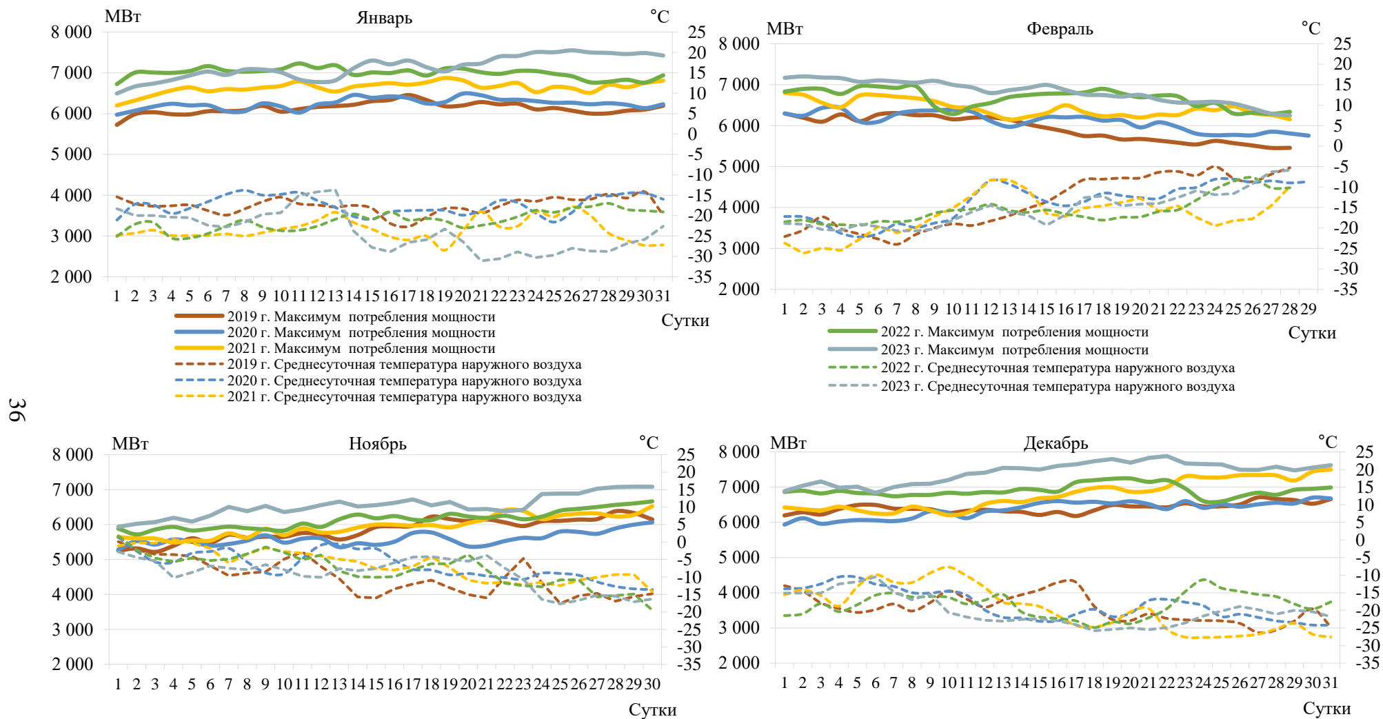
Рисунок 20 – Динамика изменения среднесуточных ТНВ и суточного максимального потребления мощности 2-й синхронной зоны ЕЭС России
