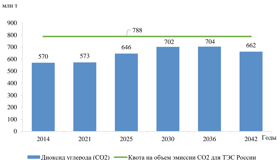
Рисунок 47 – Ожидаемые объемы эмиссии парниковых газов (диоксида углерода)
