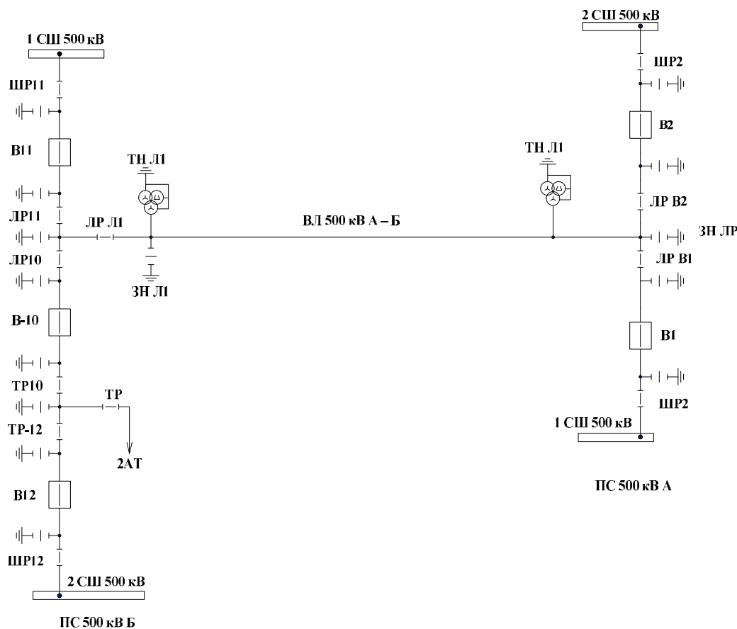
Рис. 5.1. Схема подключения ЛЭП 500 кВ А-Б
