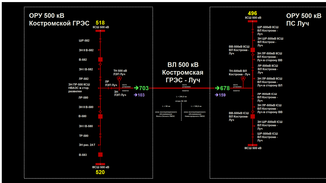
Рисунок 64. Схема ЛЭП
