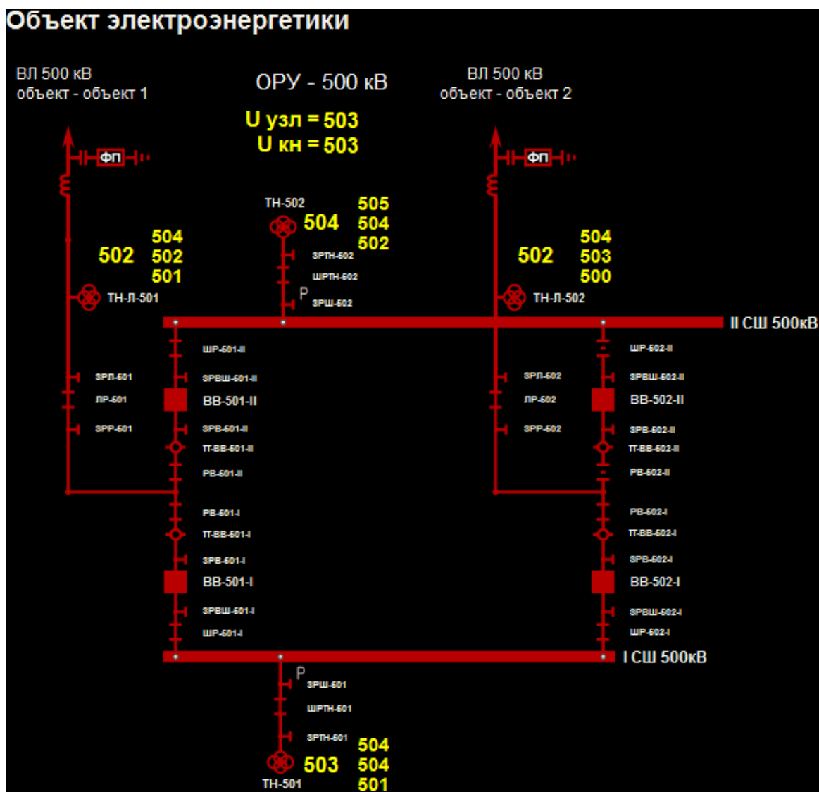
Рисунок 11. Схема ОРУ объекта ( U_{\text{ном}}=500 )
