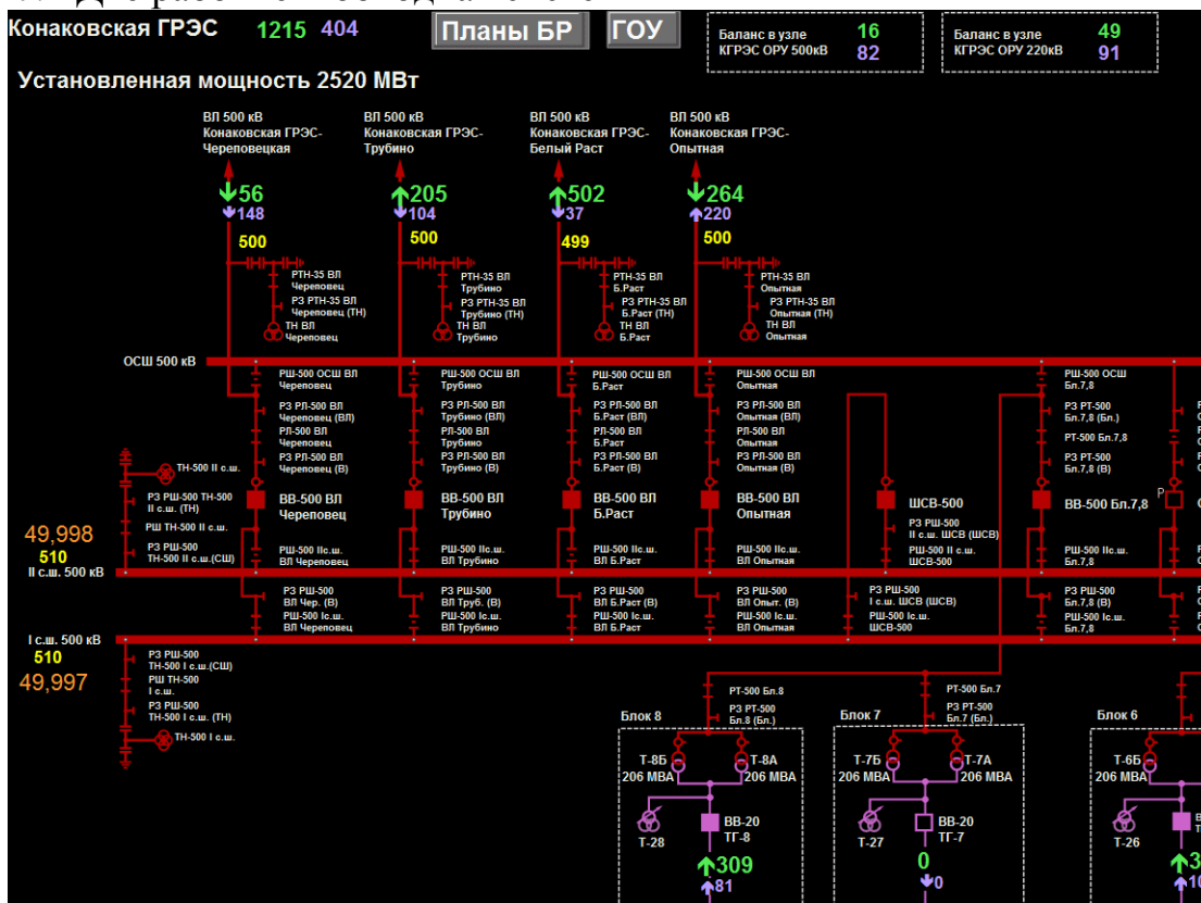
Рисунок 38. Фрагмент схемы объекта
