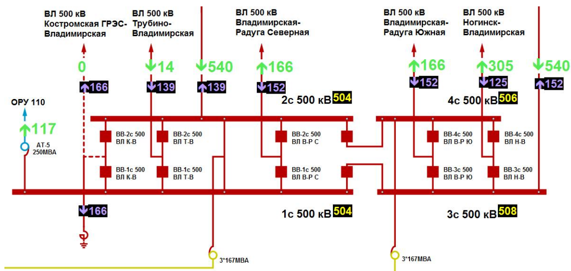
Рисунок 14. Схема ОРУ 500 кВ ПС 750 кВ Владимирская
