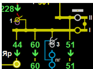
Рисунок 36. Фрагмент главной схемы
