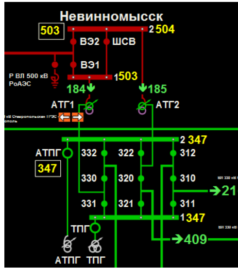
Рисунок 22. Фрагмент главной схемы
