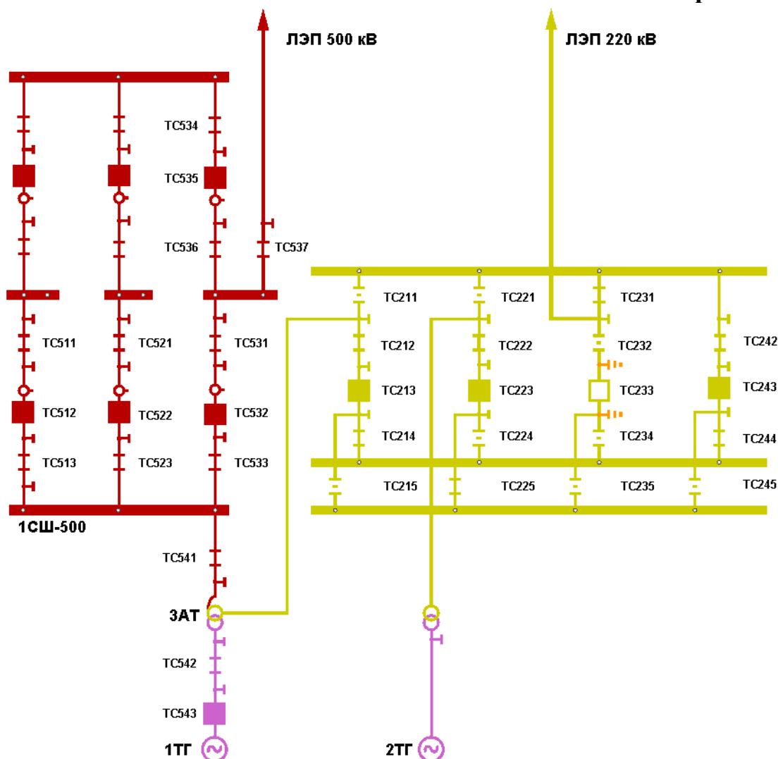
Рисунок 5. Пример схемы для описания формул ОТС
