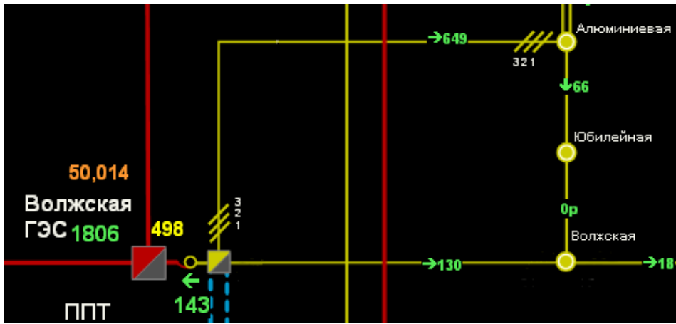
Рисунок 67. Пример режимной схемы с эквивалентной ЛЭП
