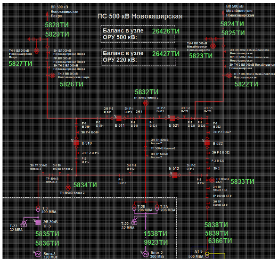
Рисунок 54. Фрагмент схемы объекта в редакторе
