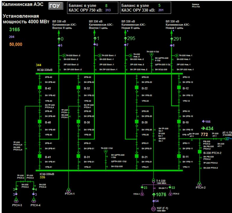
Рисунок 24. Фрагмент схемы объекта
