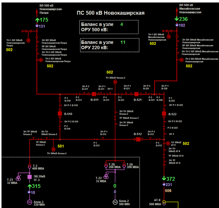
Рисунок 53. Фрагмент схемы объекта
