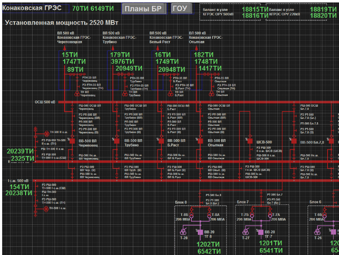
Рисунок 39. Фрагмент схемы объекта в редакторе
