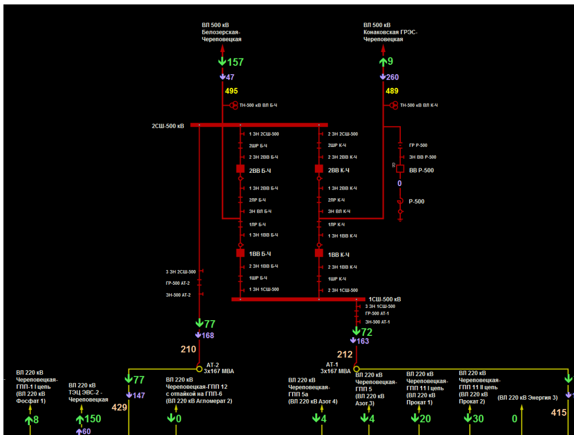
Рисунок 43. Фрагмент схемы объекта
