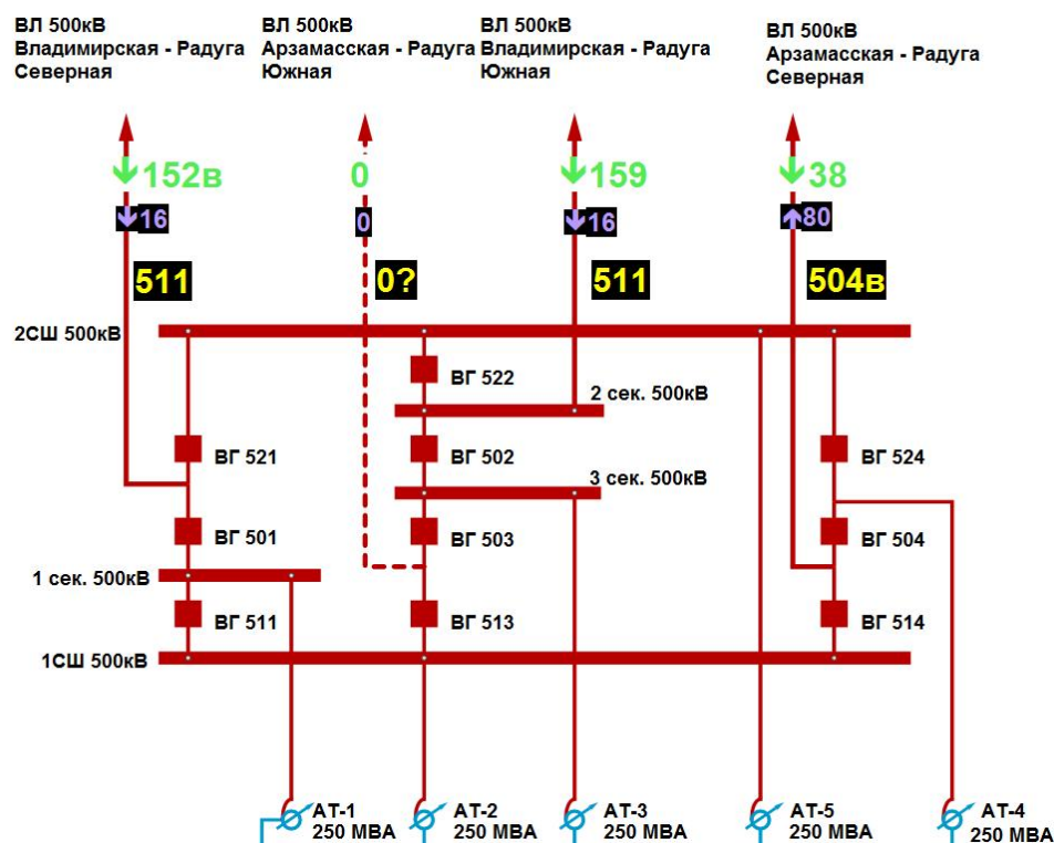
Рисунок 13. Схема объекта ПС 500 кВ Радуга
