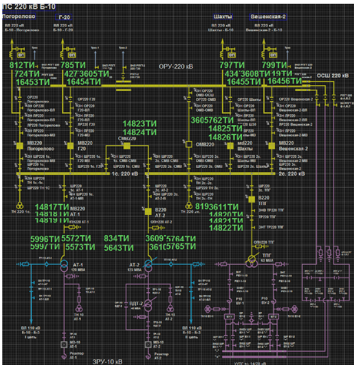
Рисунок 42. Фрагмент схемы объекта в редакторе
