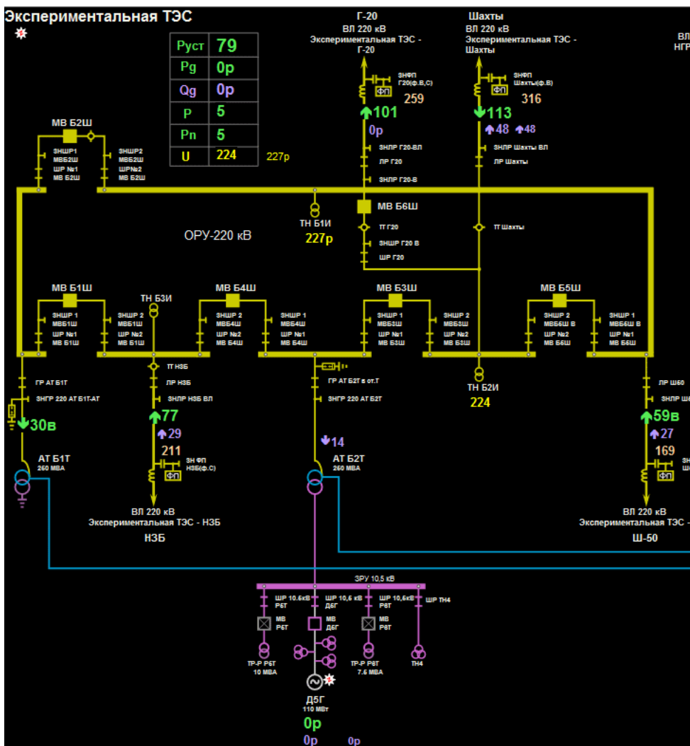
Рисунок 50. Фрагмент схемы объекта
