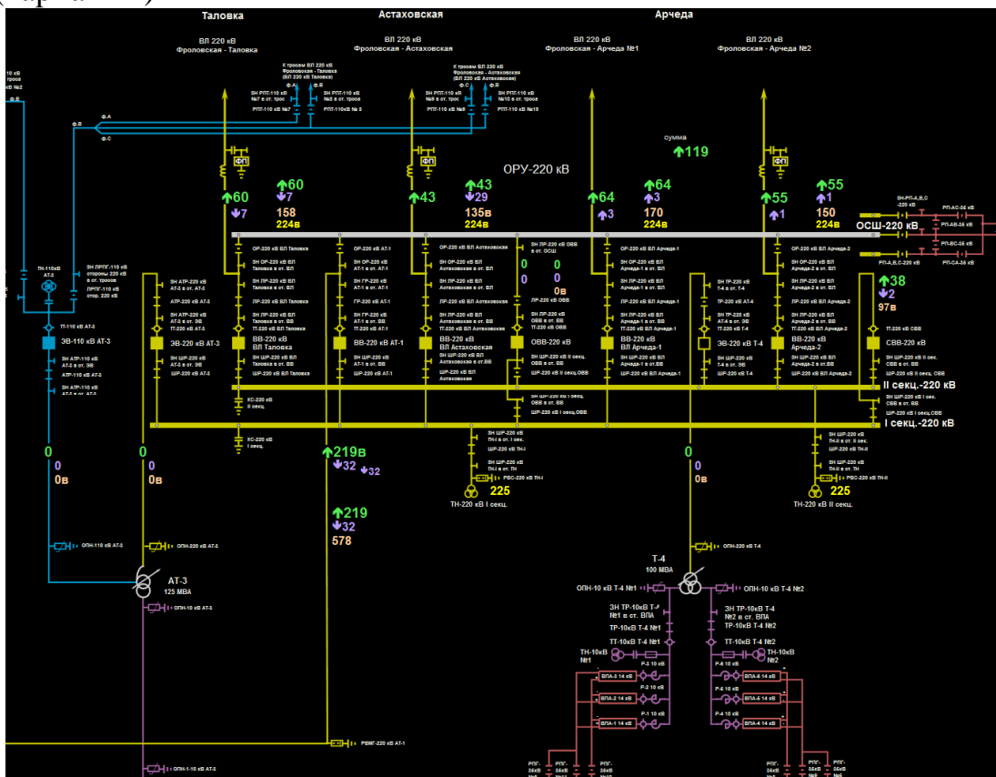
Рисунок 35. Фрагмент схемы объекта
