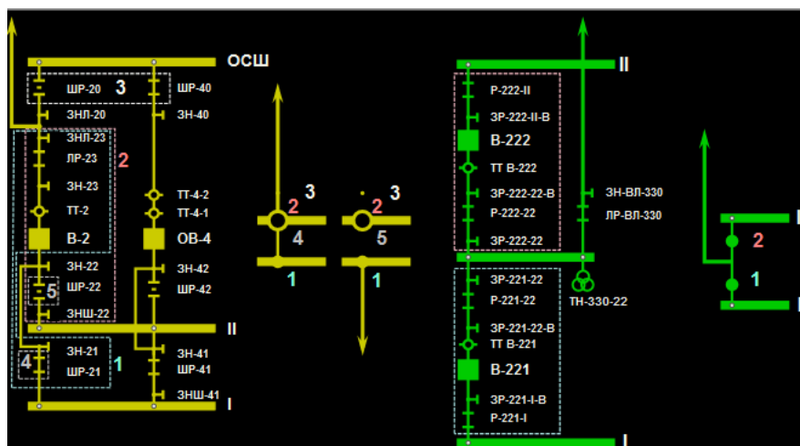
Рисунок 17. Соответствие состояний оборудования и КС
