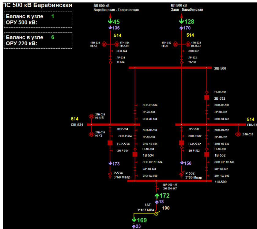
Рисунок 48. Фрагмент схемы объекта
