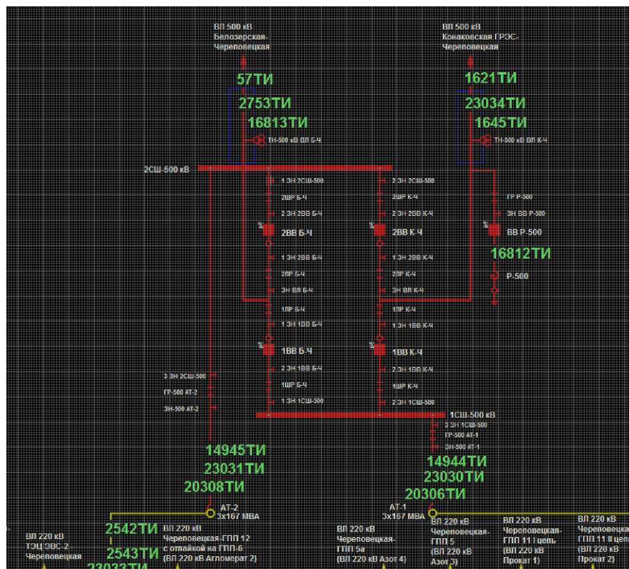
Рисунок 44. Фрагмент схемы объекта в редакторе
