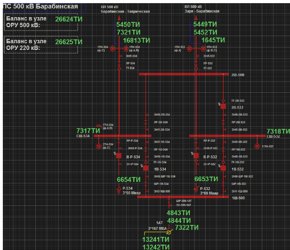
Рисунок 49. Фрагмент схемы объекта в редакторе
