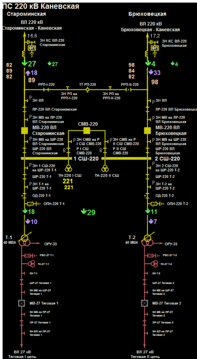
Рисунок 55. Схема объекта с отображением значений фазных токов в отключаемом слое
