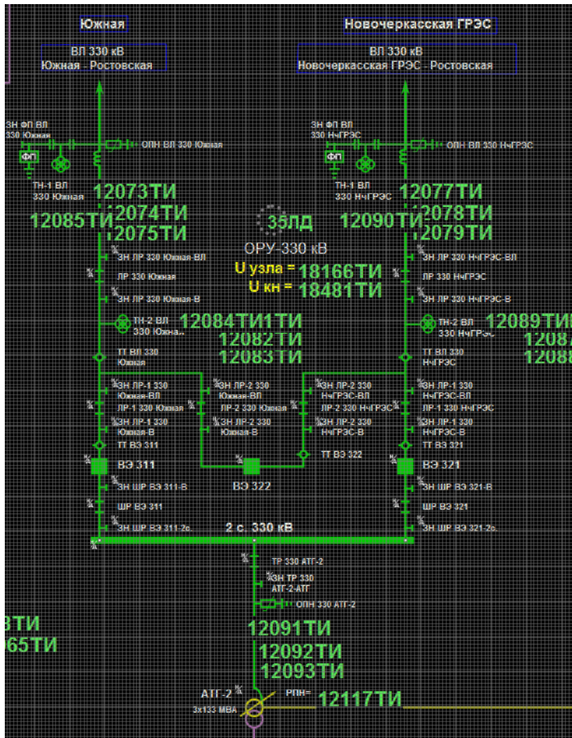
Рисунок 47. Фрагмент схемы объекта в редакторе
