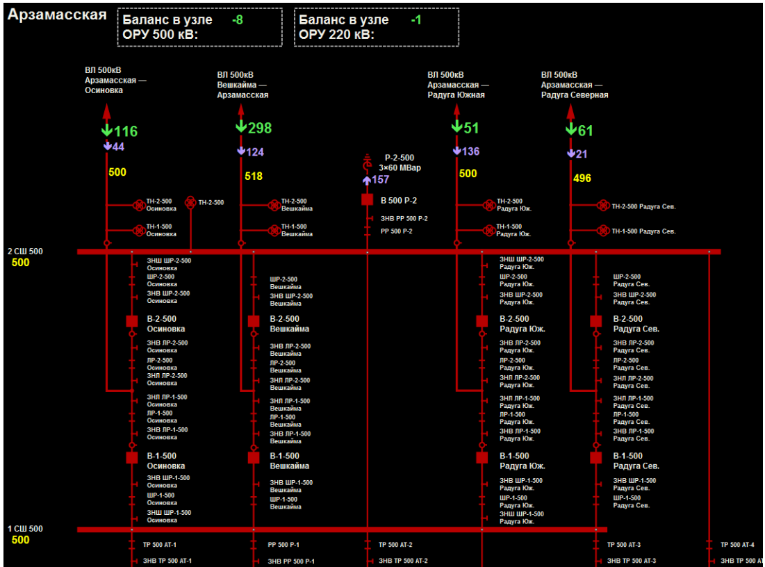
Рисунок 30. Фрагмент схемы объекта
