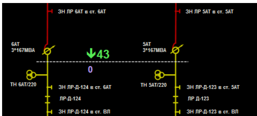
Рисунок 69. Отображение суммарных перетоков мощности по группе АТ одного класса напряжения энергообъекта со стороны СН
