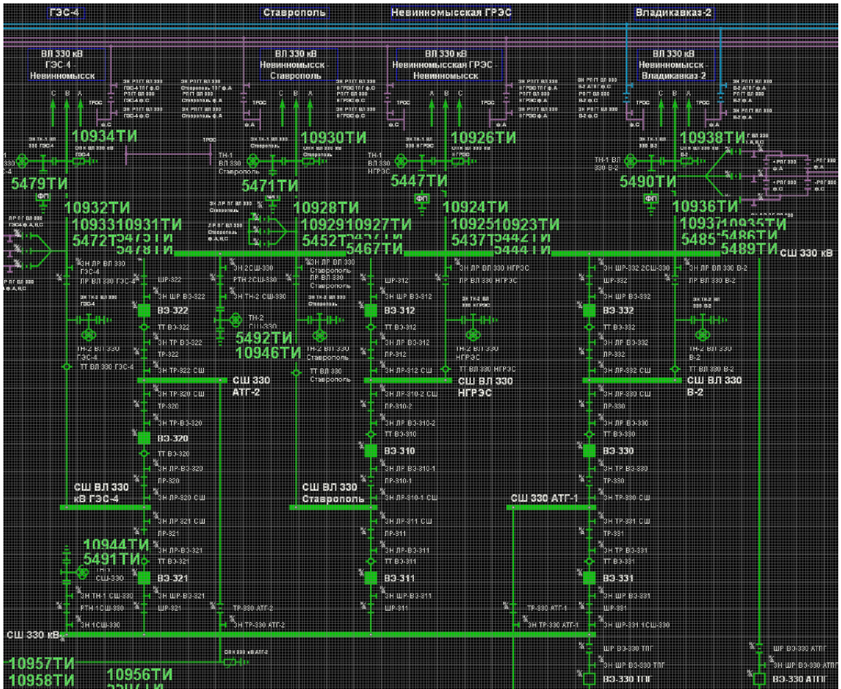
Рисунок 23. Фрагмент схемы объекта в редакторе
