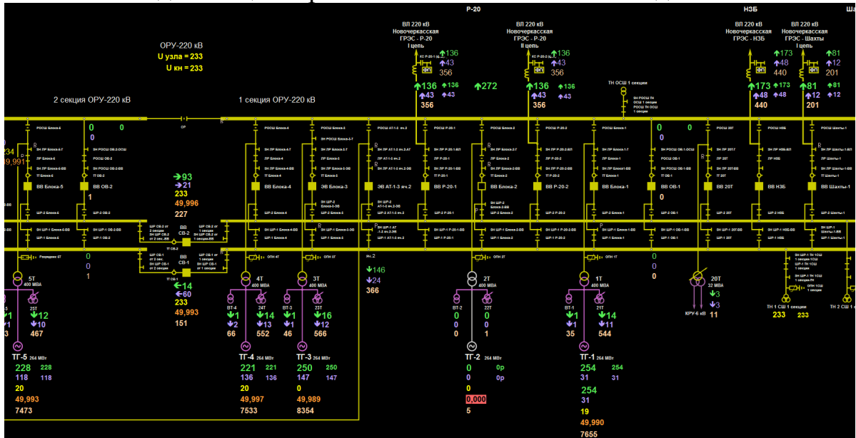
Рисунок 32. Фрагмент схемы объекта
