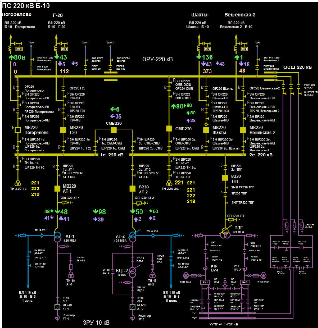
Рисунок 40. Фрагмент схемы объекта
