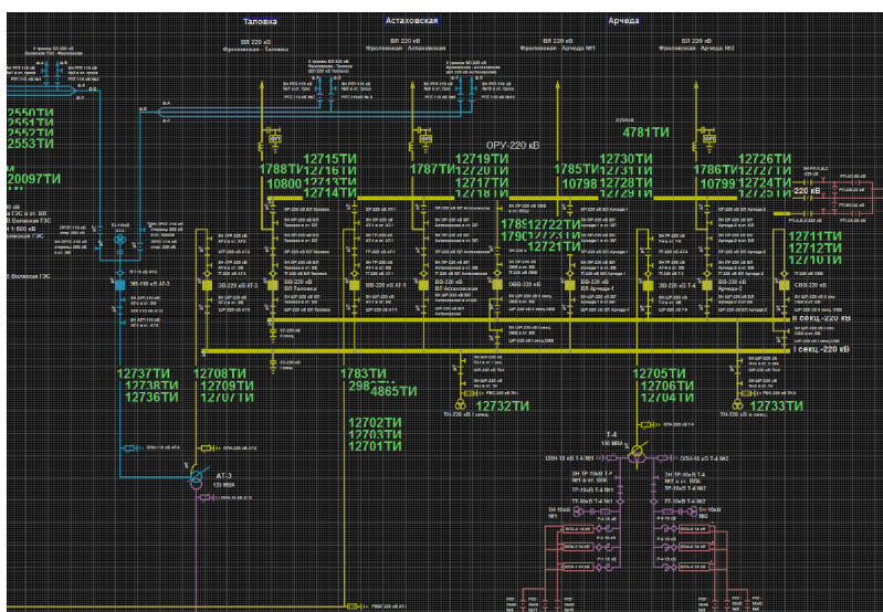
Рисунок 37. Фрагмент схемы объекта в редакторе
