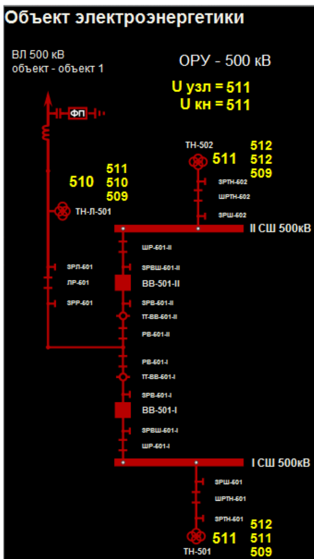
Рисунок 12. Схема ОРУ 500 кВ объекта ( U_{\text{ном}}=500 )
