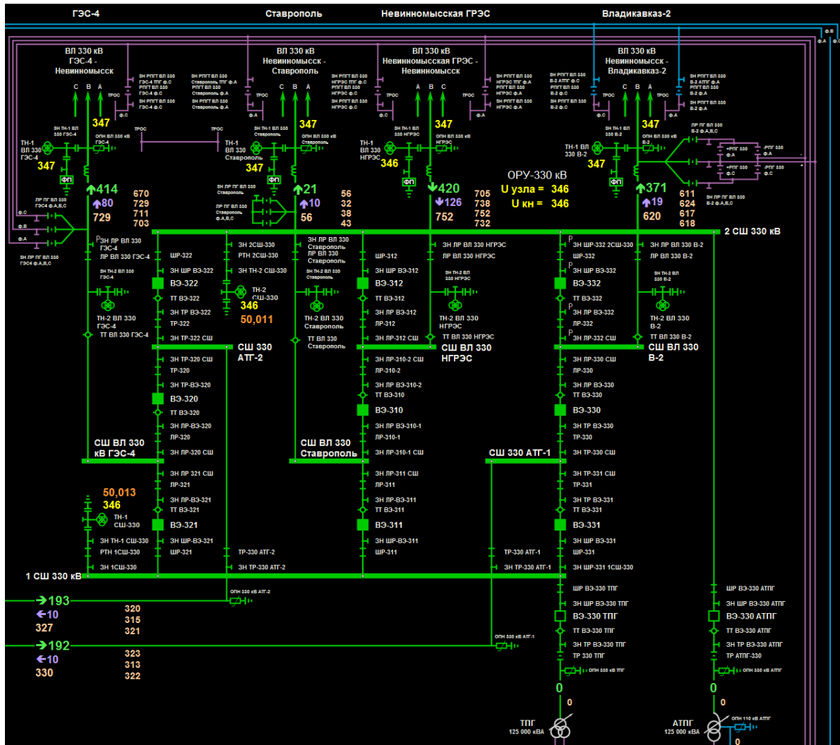
Рисунок 21. Фрагмент схемы объекта с отображением значений фазных токов в отключаемом слое
