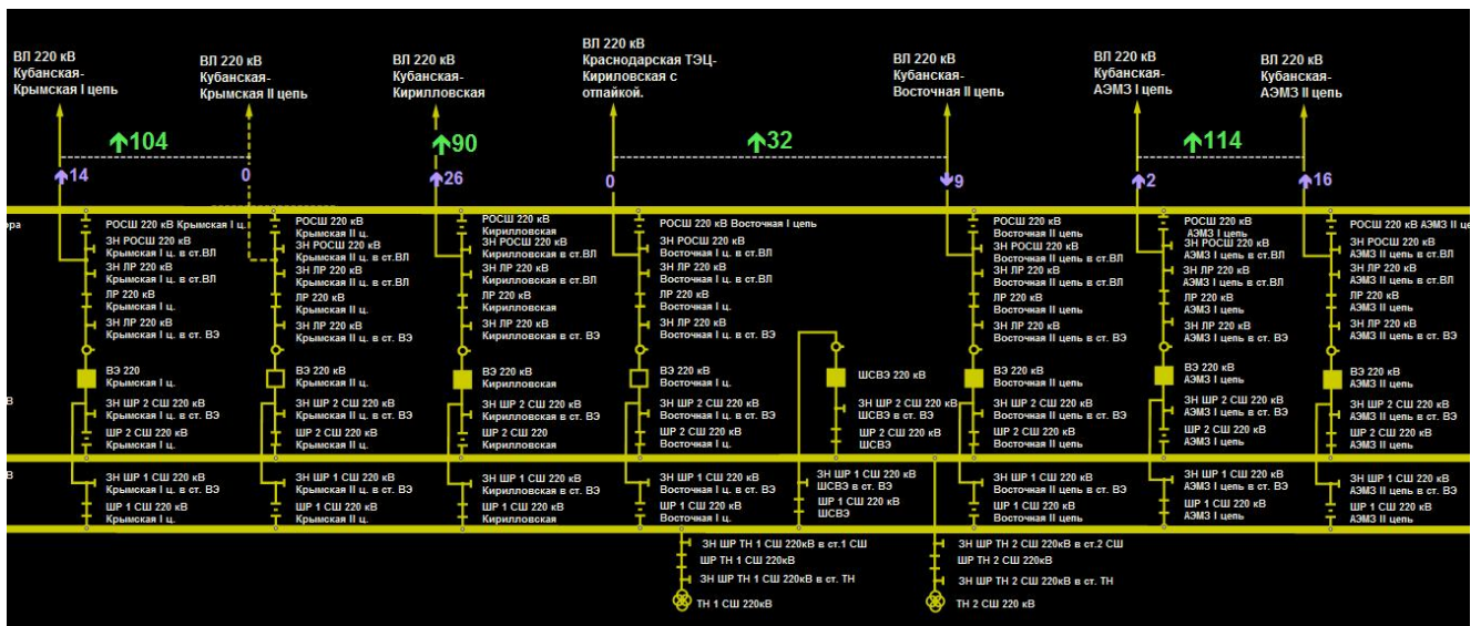
Рисунок 68. Отображение суммарных перетоков активной мощности по параллельным ЛЭП 220 кВ
