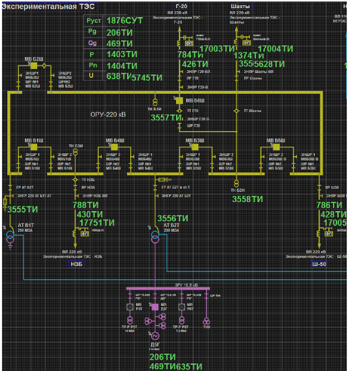
Рисунок 52. Фрагмент схемы объекта в редакторе
