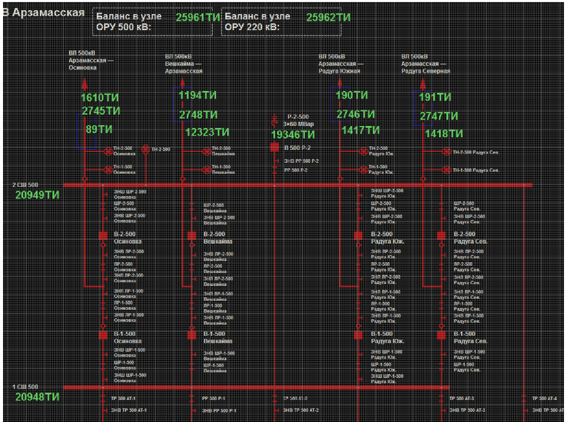
Рисунок 31. Фрагмент схемы объекта в редакторе
