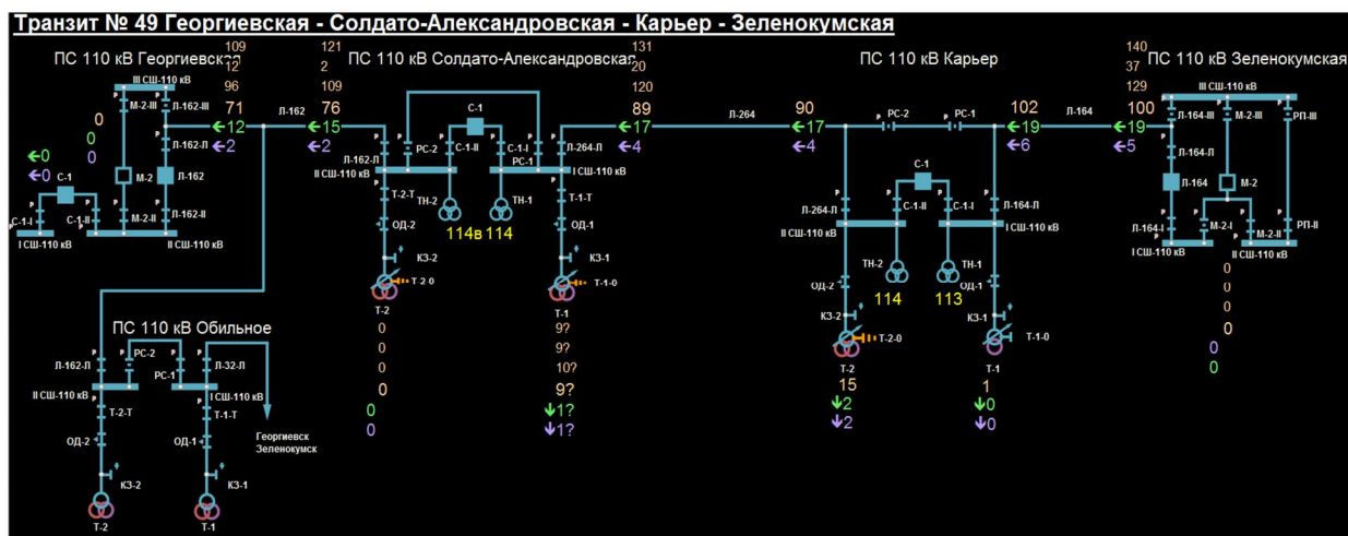
Рисунок 58. Транзит 110 кВ с отображением значений фазных токов в отключаемом слое
