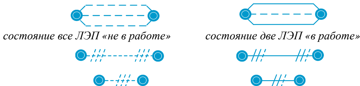
Рисунок 66. Эквивалентное исполнение нескольких линий
