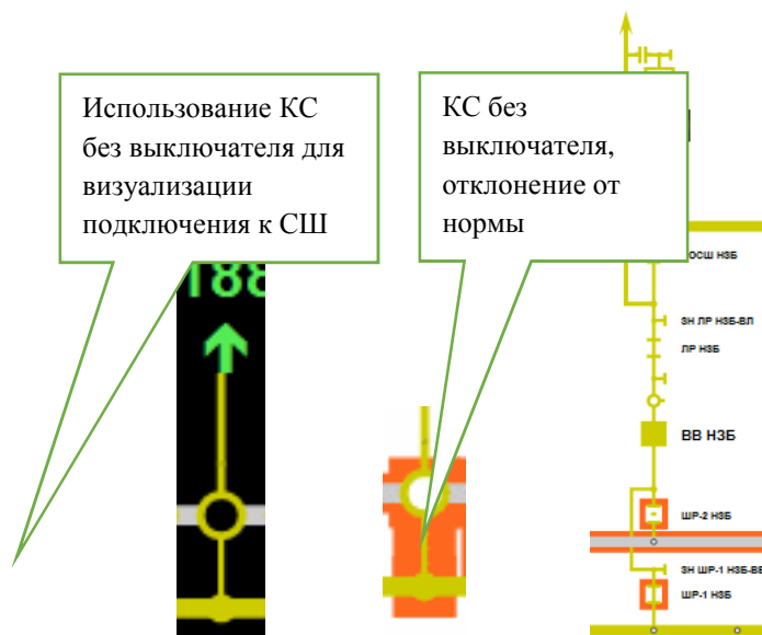
Рисунок 18. Фрагмент отображения на главной схеме и схеме объекта
