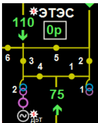
Рисунок 51. Фрагмент главной схемы
