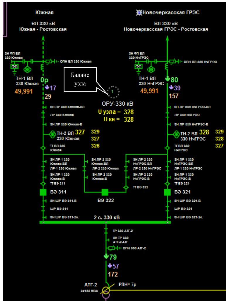
Рисунок 45. Фрагмент схемы объекта
