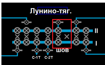
Рисунок 20. Использование КС без выключателя для шиносоединительного обходного выключателя
