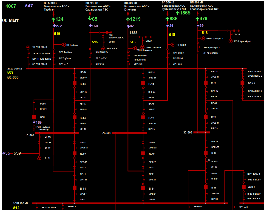
Рисунок 26. Фрагмент схемы объекта
