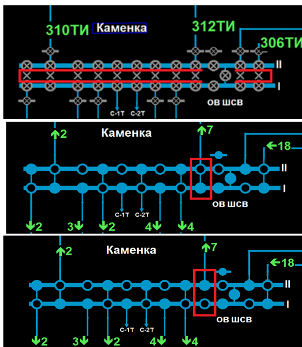
Рисунок 19. Использование КС без выключателя для визуализации присоединения к СШ
