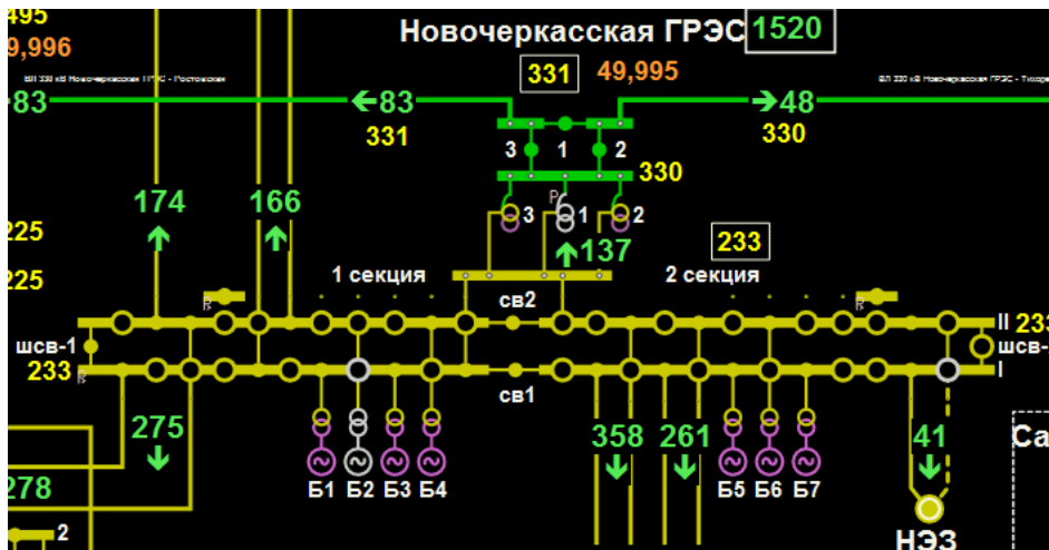
Рисунок 33. Фрагмент главной схемы
