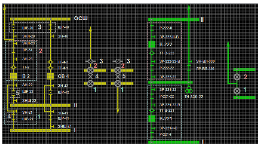
Рисунок 16. Правила формирования КС
