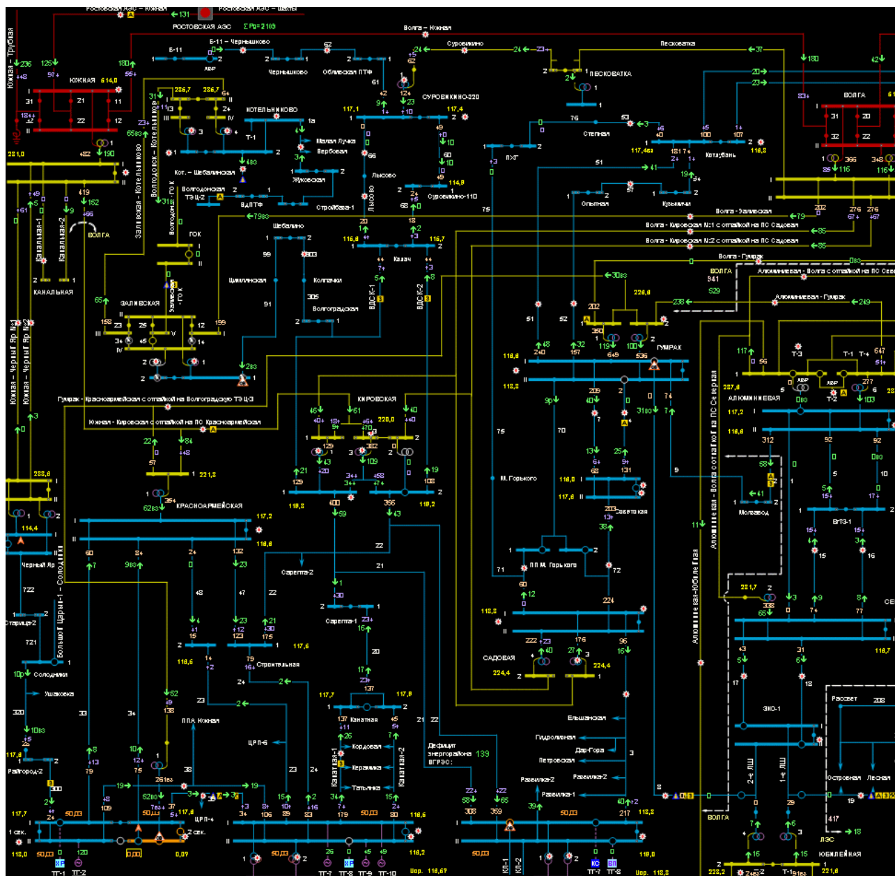
Рисунок 63. Фрагмент главной схемы
