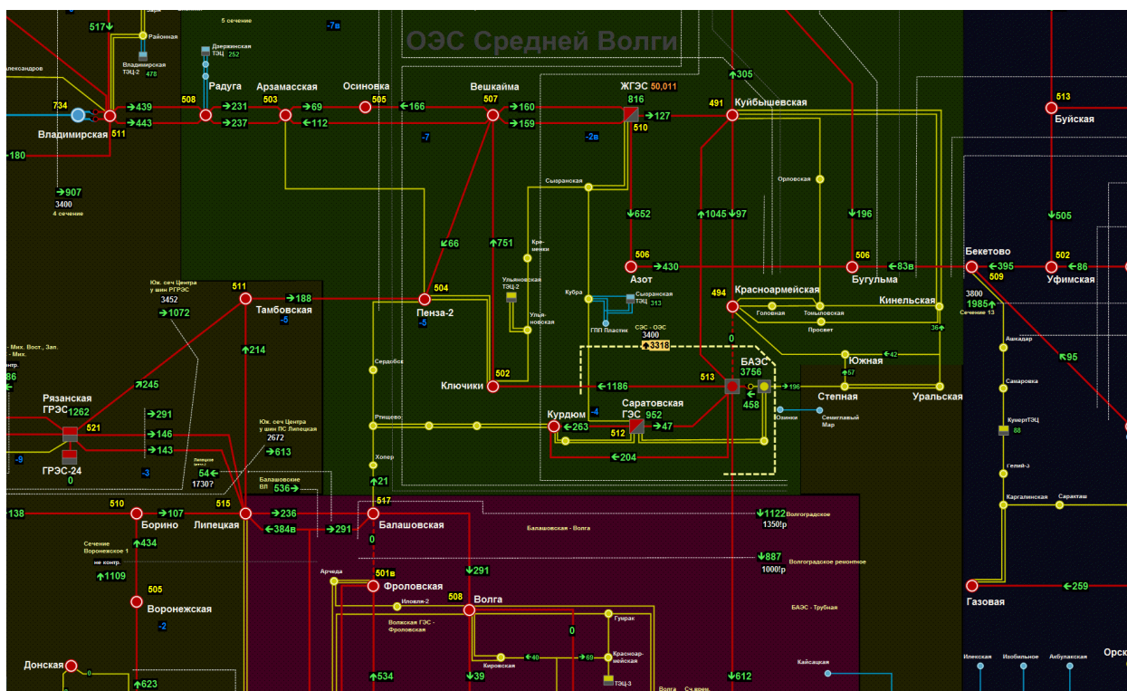
Рисунок 60. Фрагмент режимной схемы с визуализацией энергорайонов
