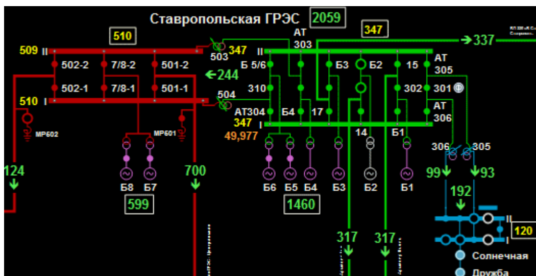
Рисунок 15. Примеры отображения напряжения в узле на схемах символического и коммутационного уровней
