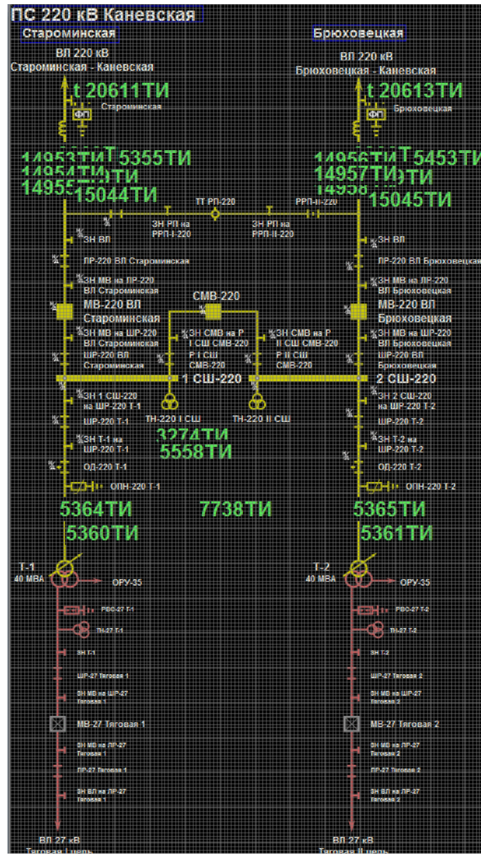
Рисунок 57. Фрагмент схемы объекта в редакторе
