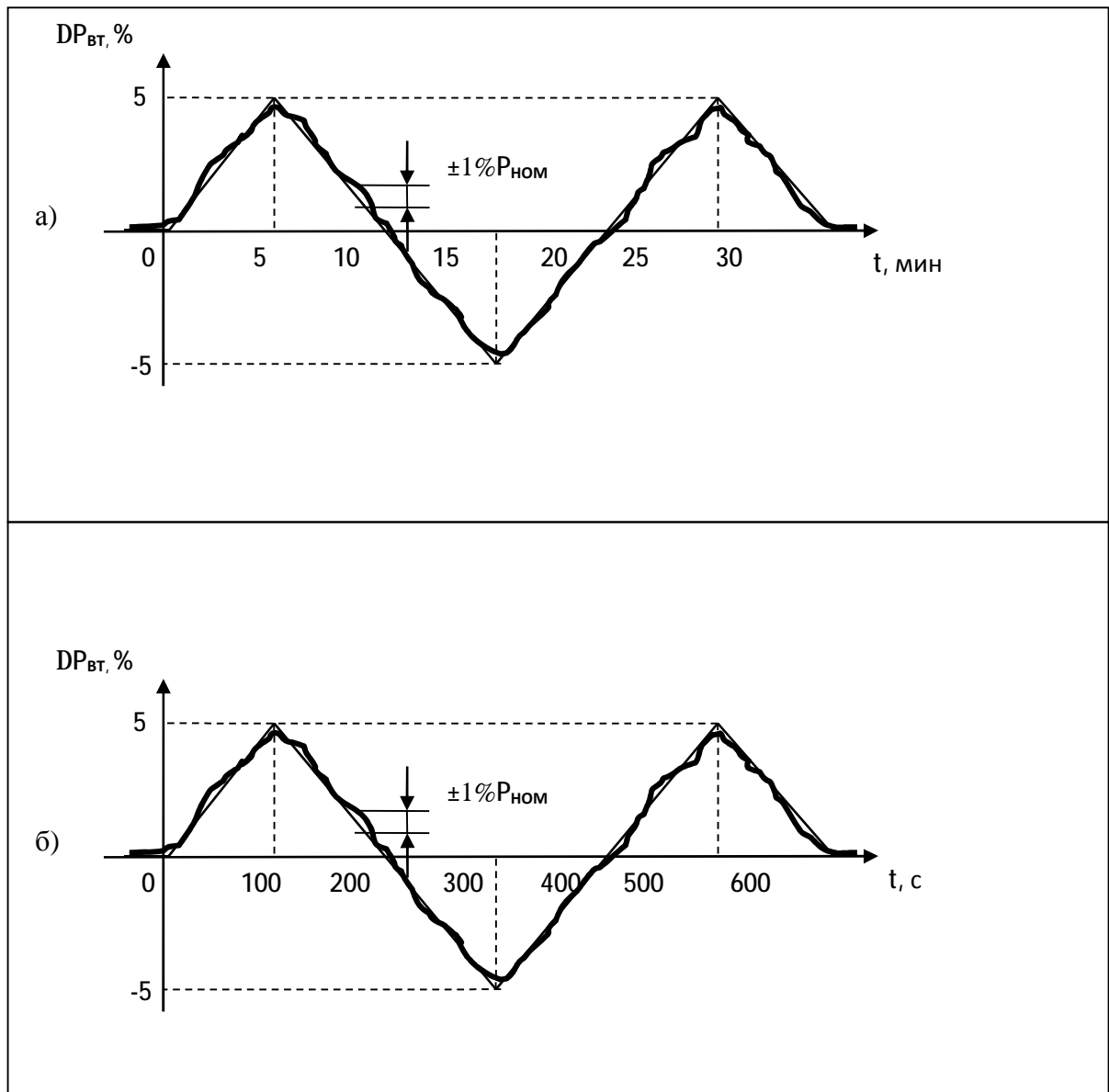
Рис.7. Имитация изменений задания и требуемые изменения вторичной мощности ПГУ при скорости задания изменения мощности 1 % P_{ном}/мин (а) и 3 % P_{ном}/мин (б)
