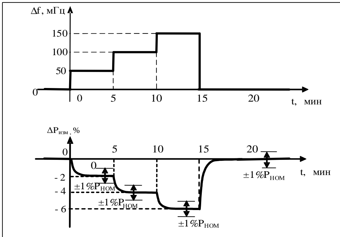
Рис. 4. Имитация повышения частоты и требуемые изменения первичной мощности ПГУ в следящем режиме
