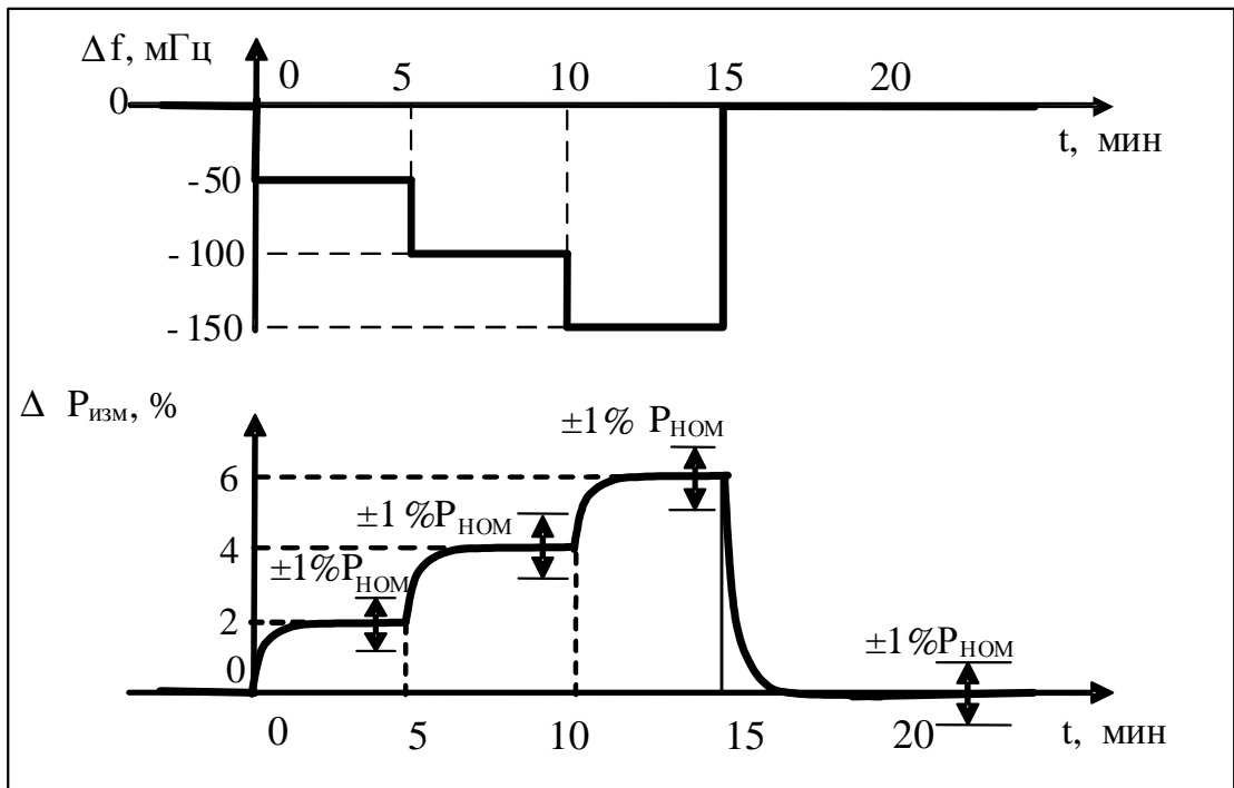
Рис. 3. Имитация снижения частоты и требуемые изменения первичной мощности ПГУ в следящем режиме
