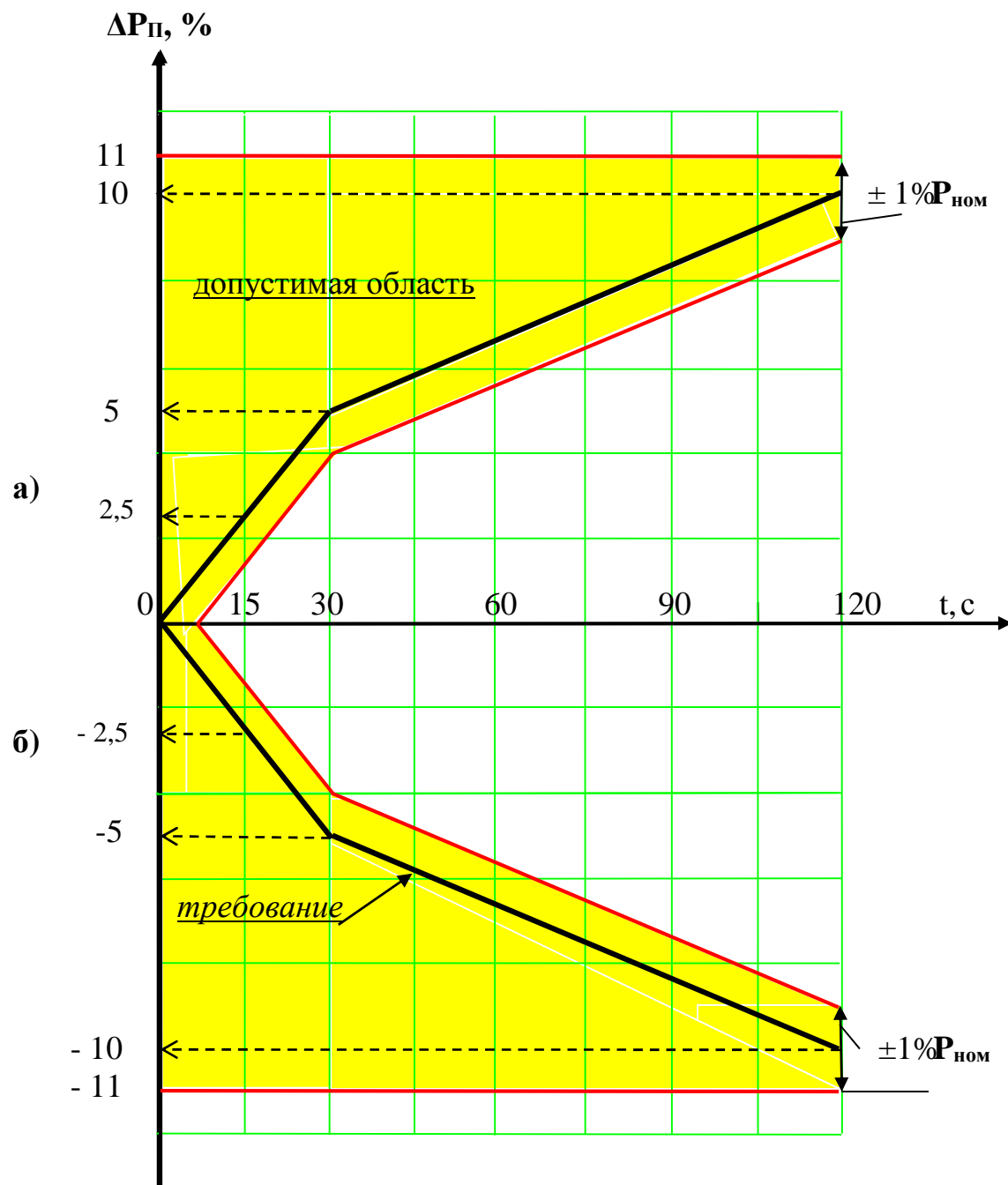
Рис. 1. Допустимая область изменения первичной мощности ПГУ при снижении (а) и повышении (б) частоты
