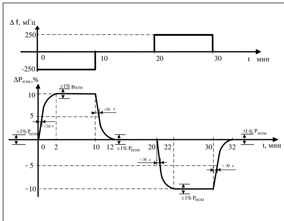
Рис. 6 Имитация отклонений частоты и требуемые изменения первичной мощности ПГУ при \Delta P_{\text{П}} = \pm 10\% P_{\text{НОМ}}
