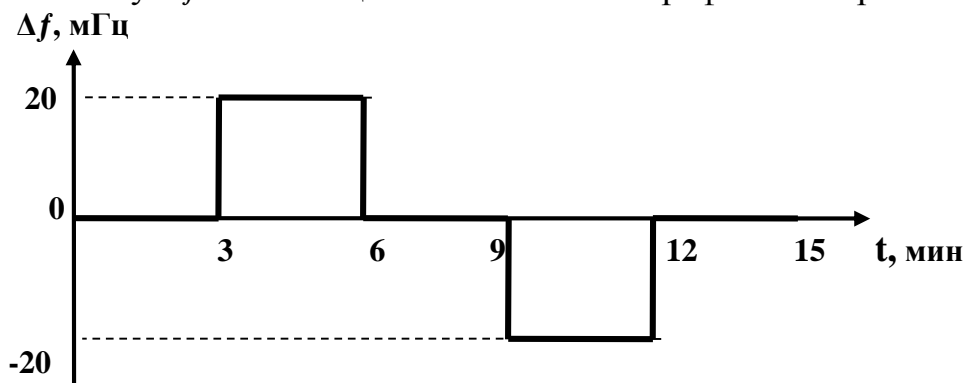
Рис. 2. Имитация отклонений частоты при проверке нечувствительности первичных регуляторов ПГУ
