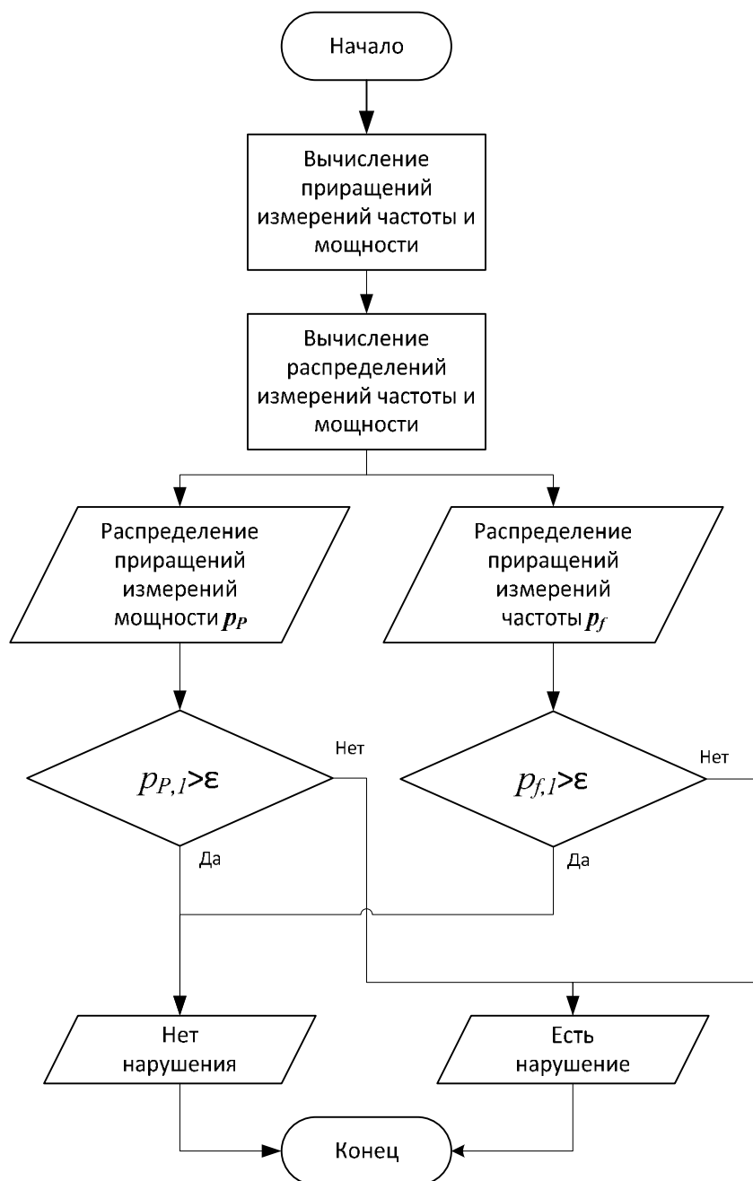
Рисунок 3. Блок-схема алгоритма "Несоответствие дискретности измерений требуемым"
