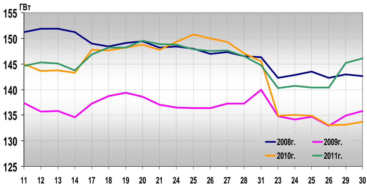
График изменения максимального потребления мощности ЕЭС России по рабочим дням января 2008-2011 годов.
