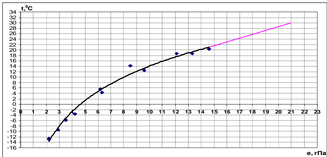
Рис. 10.1 Зависимость упругости водяного пара от температуры наружного воздуха.
