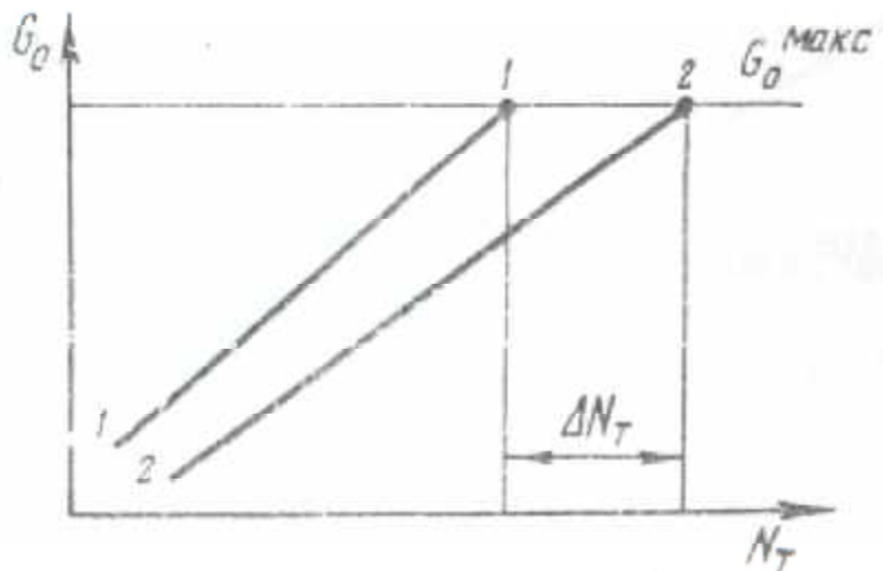
Рис. 12.6. Зависимость электрической мощности турбины типа «К» от расхода пара в голову при нормальном (линия 2-2) и ухудшенном (линия 1-1) вакууме, \Delta N – снижение мощности турбины.
