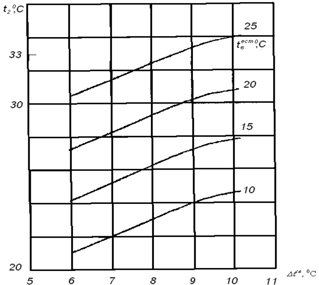
Рис. 11.8. Примерный вид зависимости t_2 = f(t_8^{ecm0}; \Delta t^{ce})
